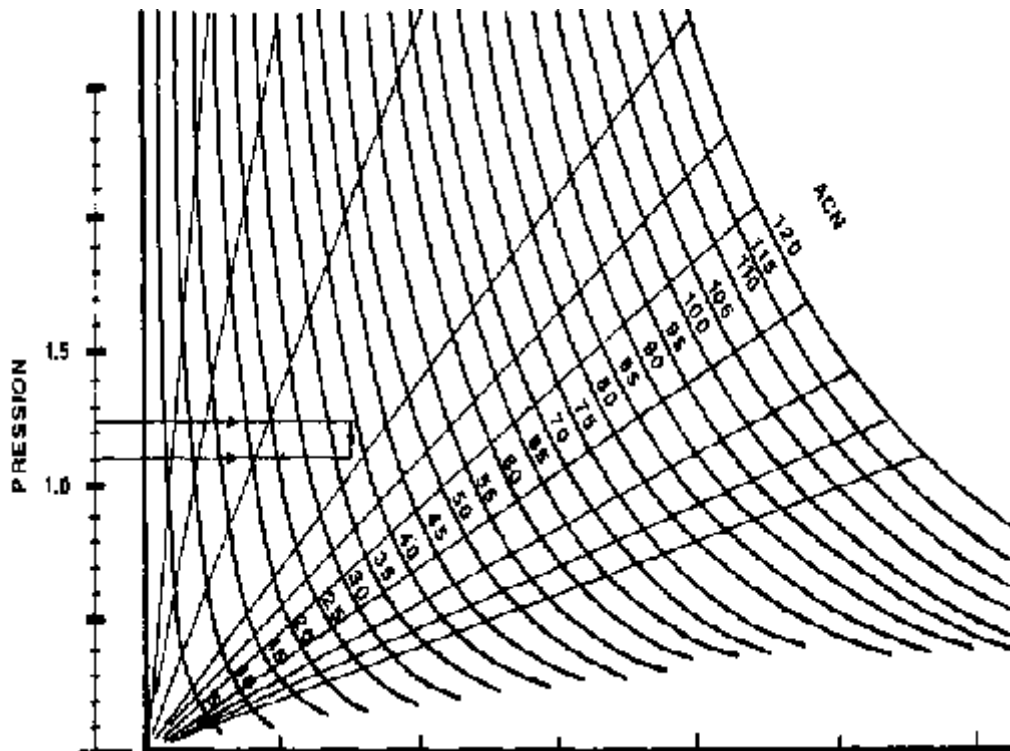
Correction des ACN en fonction de la pression réelle q' de gonflage des pneumatiques sur chaussée rigide
