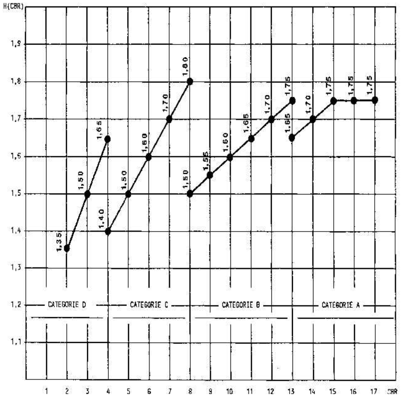
FIGURE 2 : Valeurs du coefficient H(CBR) pour le calcul du PCN approché sur chaussées souples
