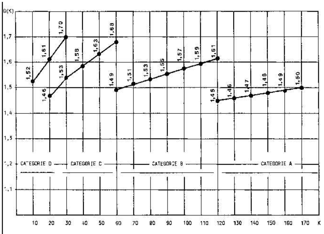
FIGURE 3 : Valeurs du coefficient G (K) pour le calcul du PCN approché sur chaussées rigides
