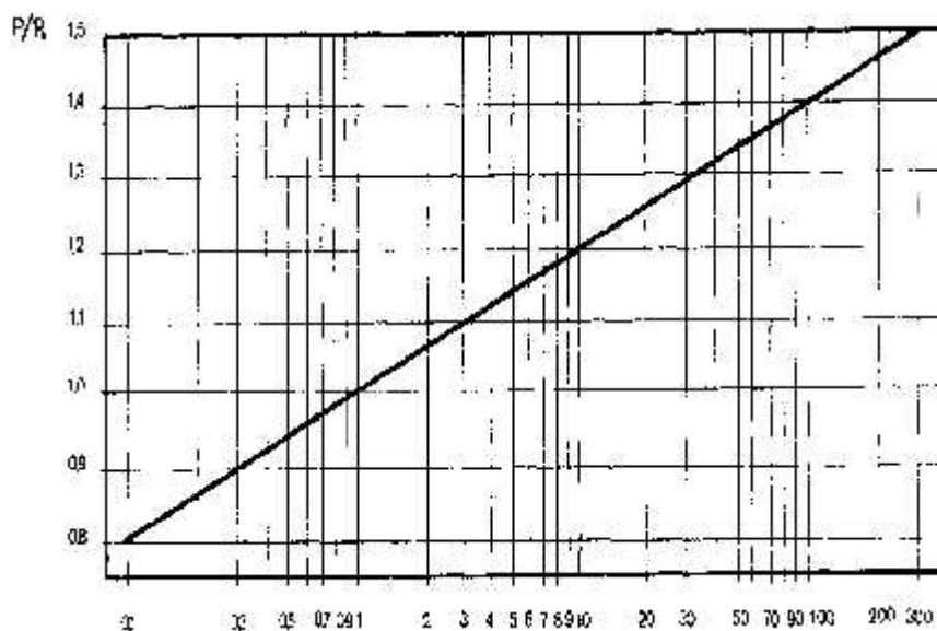
Figure 4 : Abaque pour la pondération des mouvements réels
