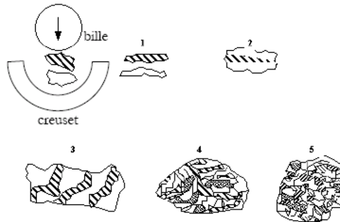
Figure 1.2 : Schéma de principe du broyage à haute énergie : alternance de déformations plastiques, fractures, collages [9].
