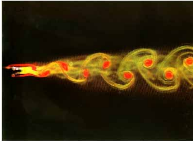
FIGURE 2.2 – Tourbillons générés suite à l'écoulement autour d'une plaque plane (www.effluids.com)
