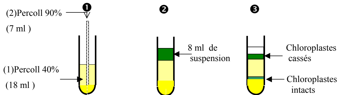
Figure 2.4 : les étapes de la séparation des chloroplastes intacts en utilisant un gradient du percoll:
