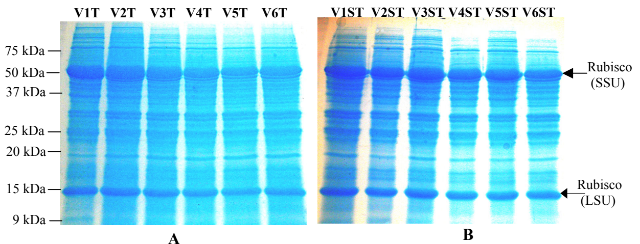
Figure 3.5 : Profils SDS-PAGE révélés au bleu de Coomassie de protéines foliaires solubles de plantes d'orge Hordeum vulgare témoins et soumises à un déficit hydrique de 8 jours au stade tallage.
