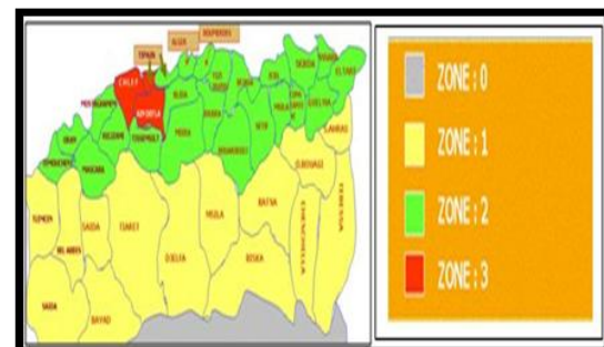
Figure III.16: La classification de la sismicité de la ville de Tipaza. Source : Fr.wikipedia.com
