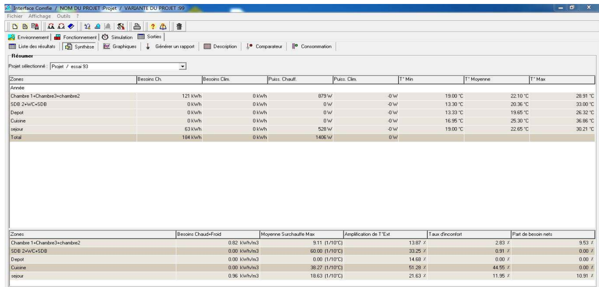
Figure III .34: besoin et puissance de chauffage en hiver
