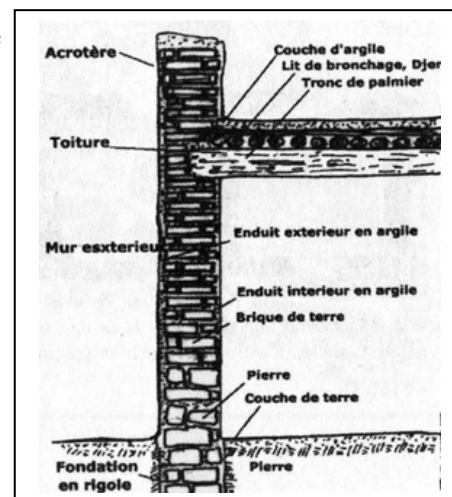
Figure III.09: Matériaux et système Constructif
