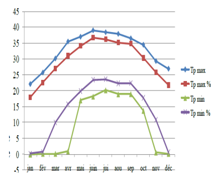
Graph III.3 variation de température
