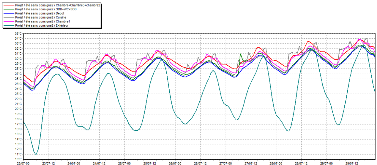
Figure III.33: variation des températures de la période estivale sans consigne.
