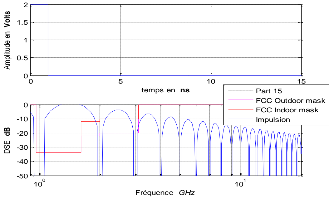
Figure 4.3 : Représentation temporelle et spectrale de l'impulsion rectangulaire.
