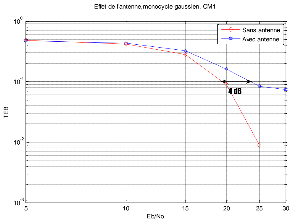
Figure 4.23 : la comparaison de performances entre le système implémentant des antennes d'émission et celui sans antennes.
