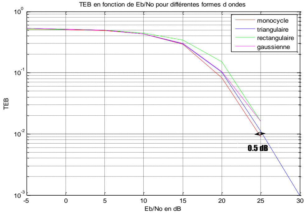
Figure 4.21 : TEB en fonction de E_b/N_0 pour différentes formes d'ondes.
