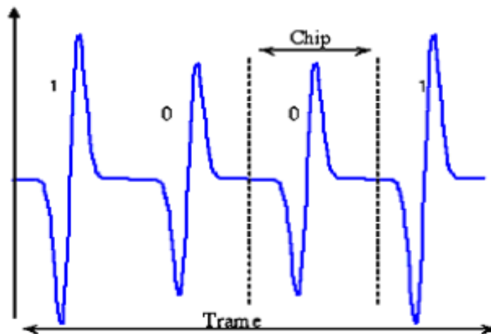
Figure 2.6 : Modulation d'impulsion en amplitude.
