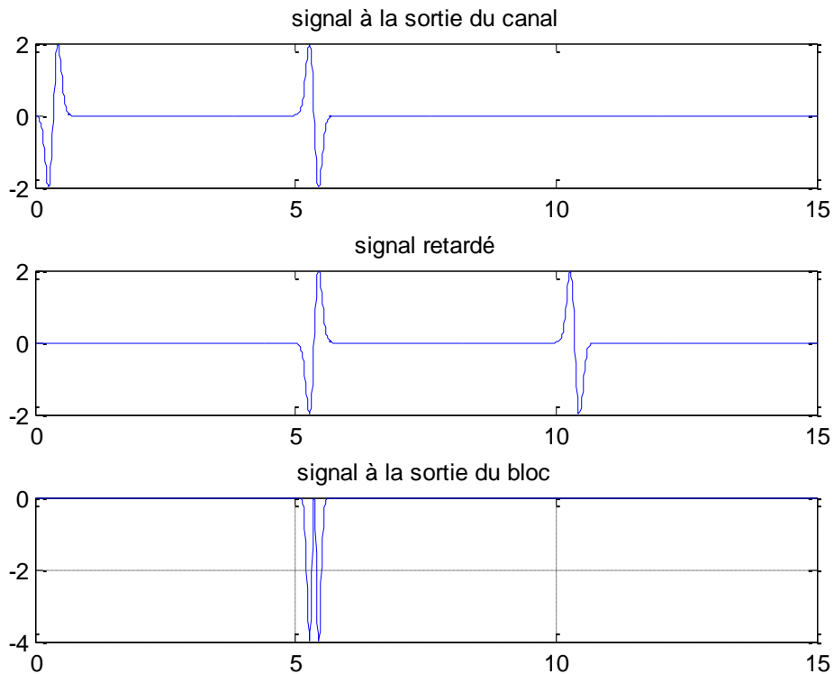
Figure 3. 6 : Retard et multiplication dans le cas d'une transmission d'un « 0 ».
