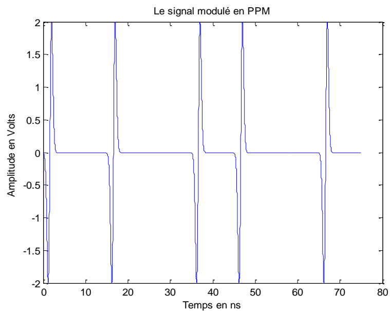
Figure 4.7 : La séquence modulée en PPM.
