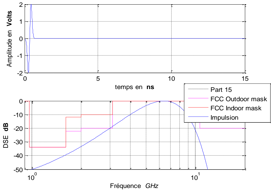
Figure 4.2 : Représentation temporelle et spectrale du monocycle gaussien.
