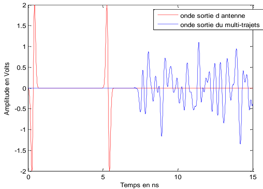
Figure 4.13 : Convolution du premier dans le canal.
