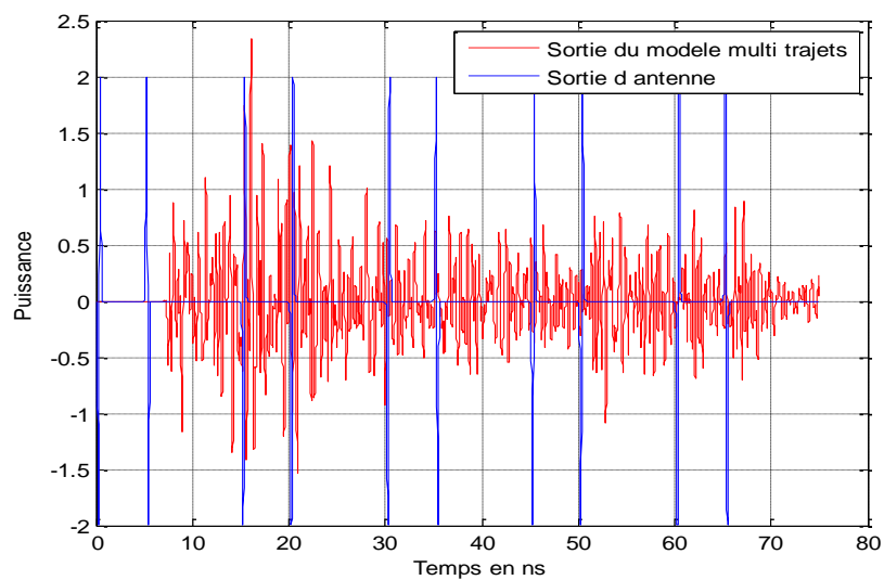
Figure 4.14 : Passage de la séquence entière à travers le canal.
