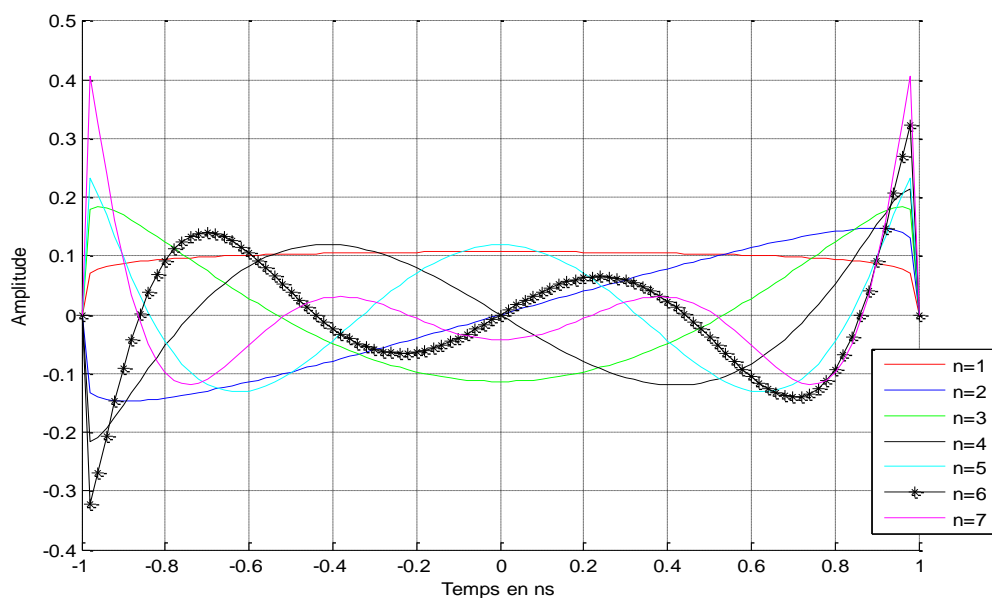
Figure 3.8 : Représentation temporelle pour les 7 premiers ordres de Gegenbauer pour \beta=1
