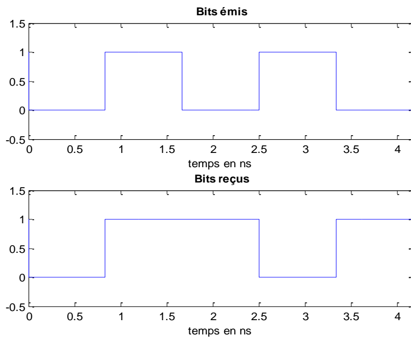
Figure 4.12: Bits émis / Bits reçus.
