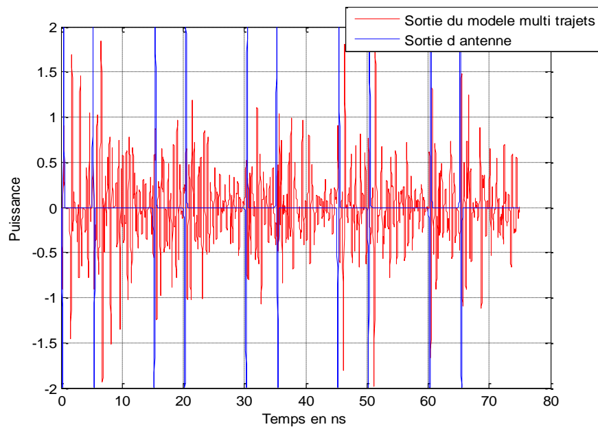
Figure 4.9 : Passage de la séquence entière à travers le canal.
