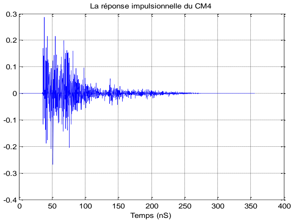
Figure 2.14 : Réalisations des 4 canaux du modèle IEEE 802.15.3a.
