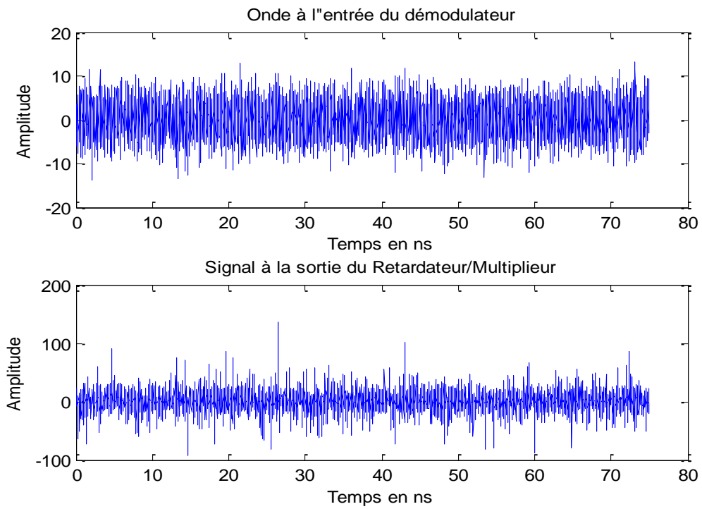
Figure 4.11 : Onde à l'entrée et à la sortie du multiplicateur/retardateur.
