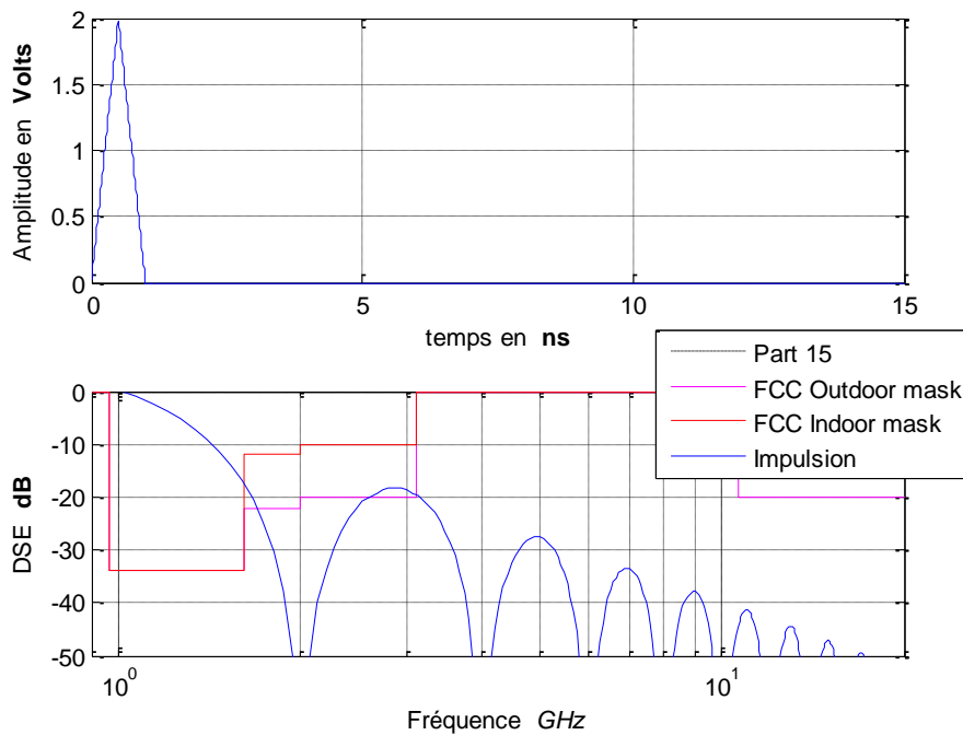
Figure 4.4 : Représentation temporelle et spectrale de l'impulsion triangulaire.
