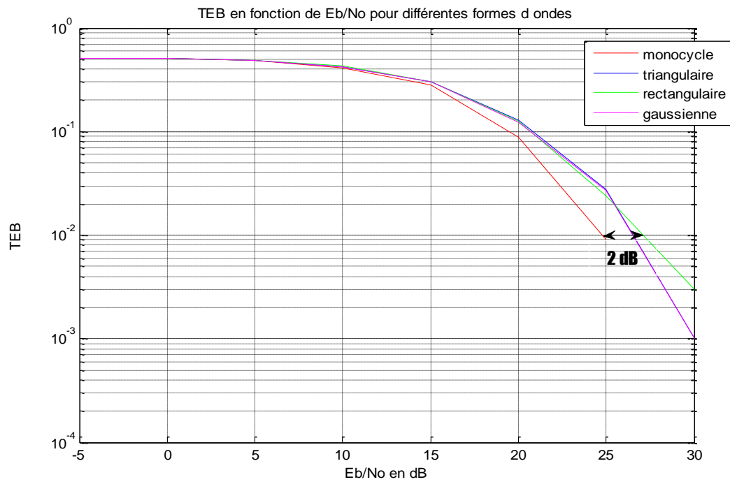
Figure 4.18 : TEB en fonction de Eb/No pour différentes formes d'ondes.
