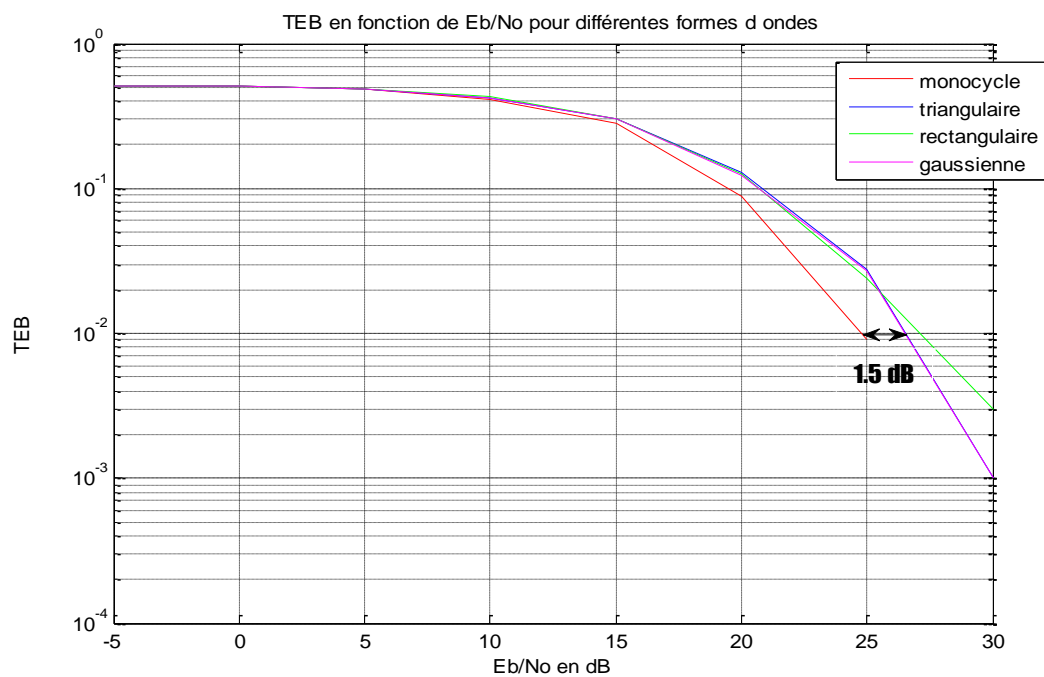
Figure 4.19 : TEB en fonction de Eb/No pour différentes formes d'ondes.
