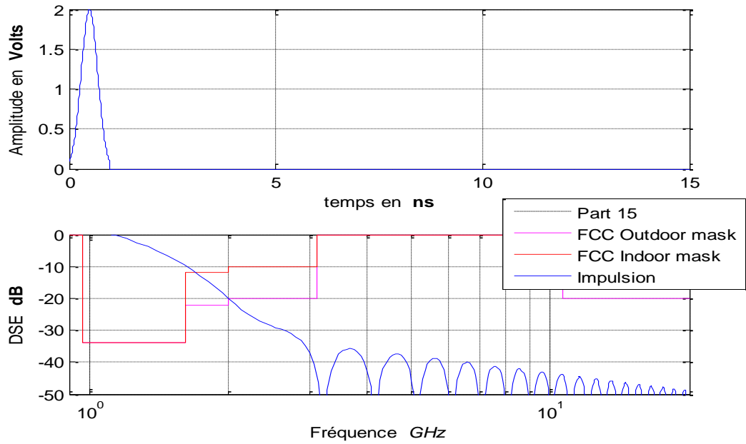
Figure 4.1 : Représentation temporelle et spectrale de l'impulsion gaussienne.
