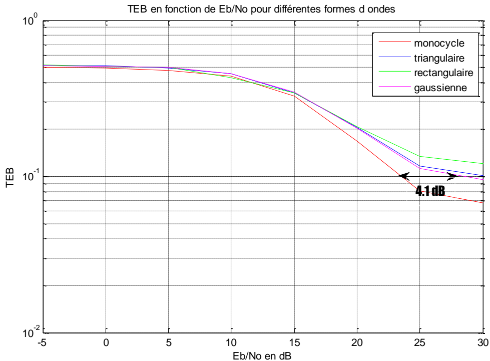
Figure 4.20 : TEB en fonction de Eb/No pour différentes formes d'ondes.
