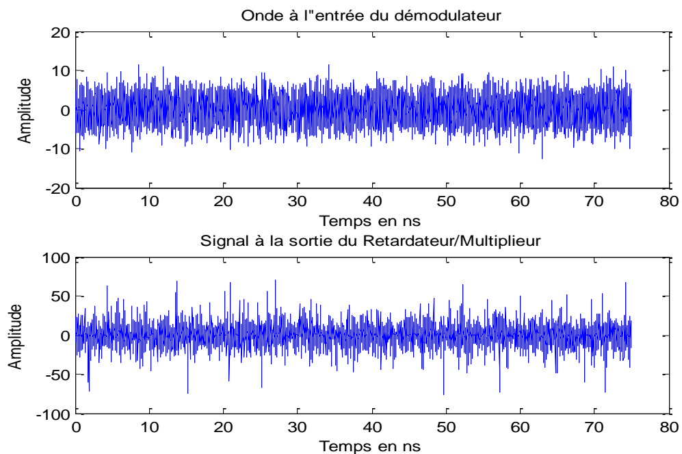
Figure 4.16 : Onde à l'entrée et à la sortie du multiplicateur/retardateur.
