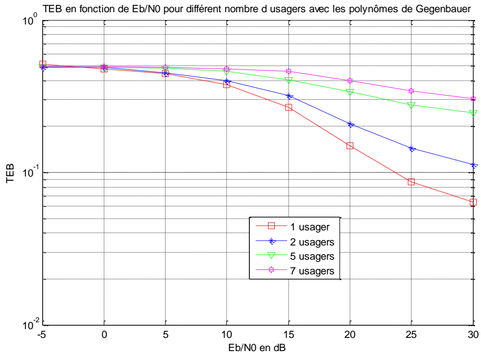
Figure 4.25 : TEB en fonction de E_b/N_0 pour différent nombre d'usagers avec les polynômes de Gegenbauer.
