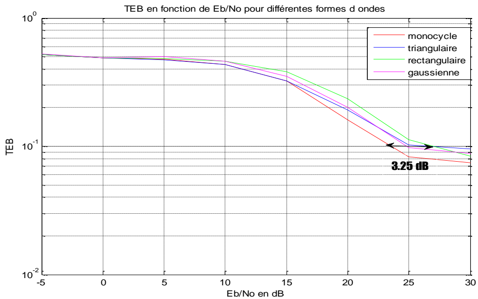
Figure 4.22 : TEB en fonction de E_b/N_0 pour différentes formes d'ondes.
