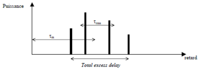
Figure 2.13 : Illustration des caractéristiques du profil de puissance.
