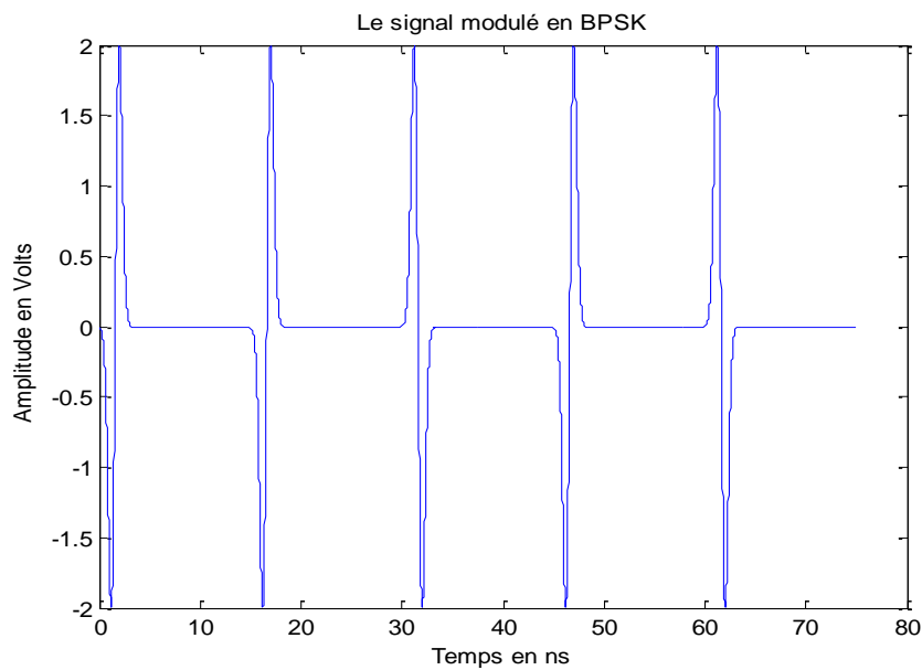
Figure 4.5 : La séquence modulée en BPSK.
