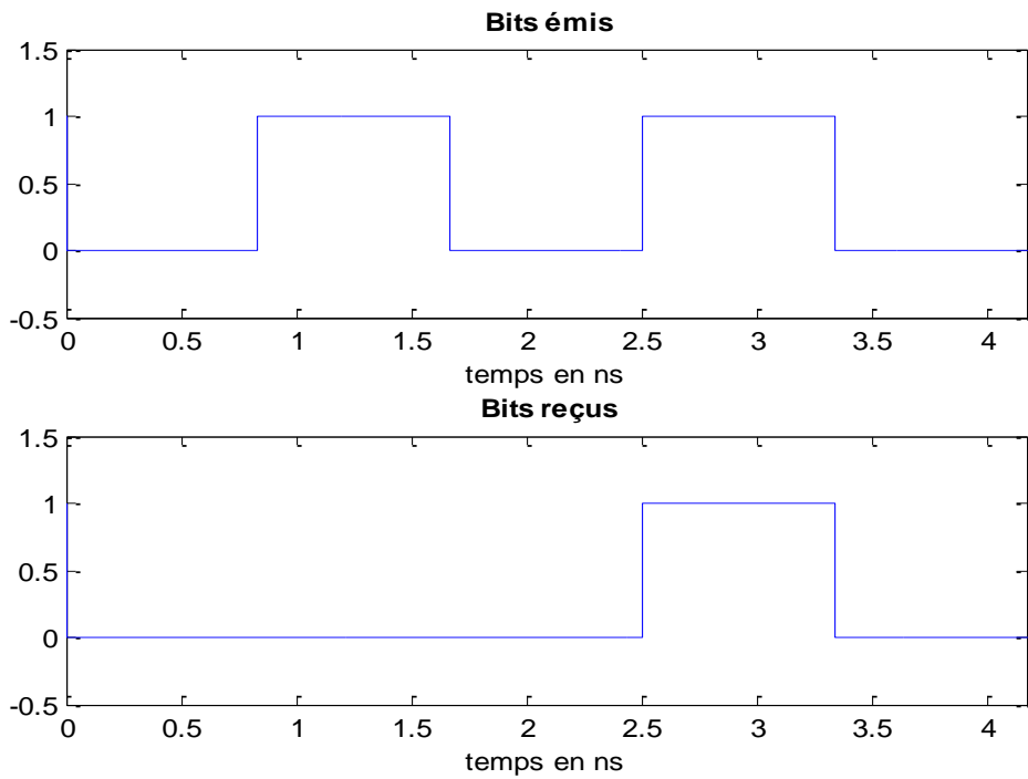
Figure 4.17 : Bits émis / Bits reçus.
