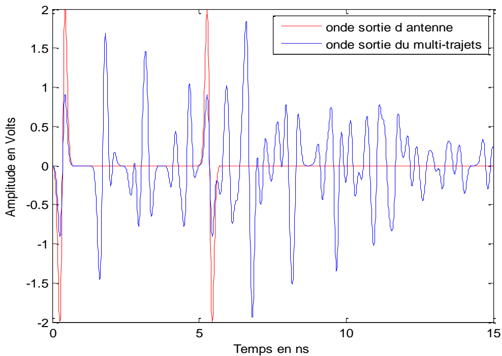
Figure 4.8 : Convolution du premier bit avec le canal.
