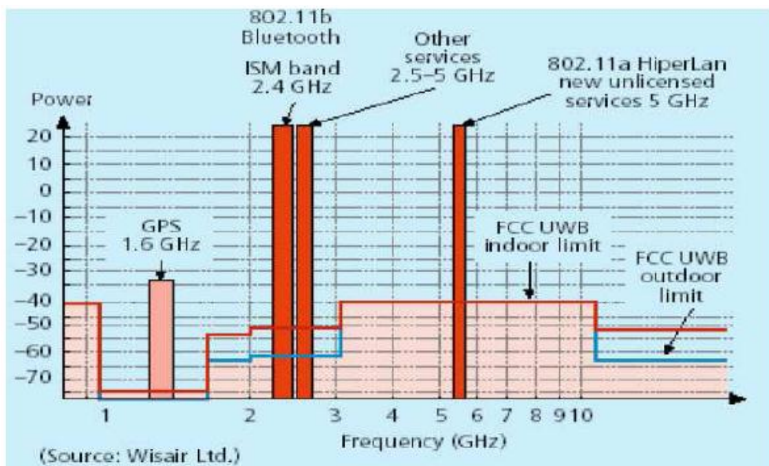
Figure 1.4 : Spectre des différents systèmes qui coexistent avec l'ULB.
