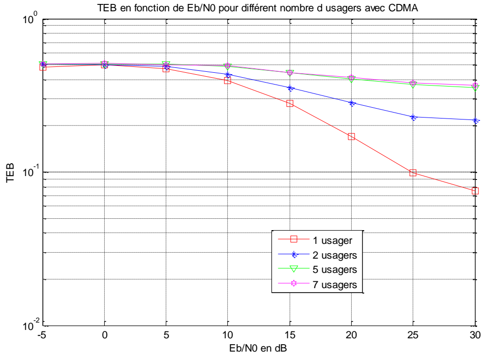
Figure 4.24 : TEB en fonction de E_b/N_0 pour différent nombre d'usagers avec CDMA.
