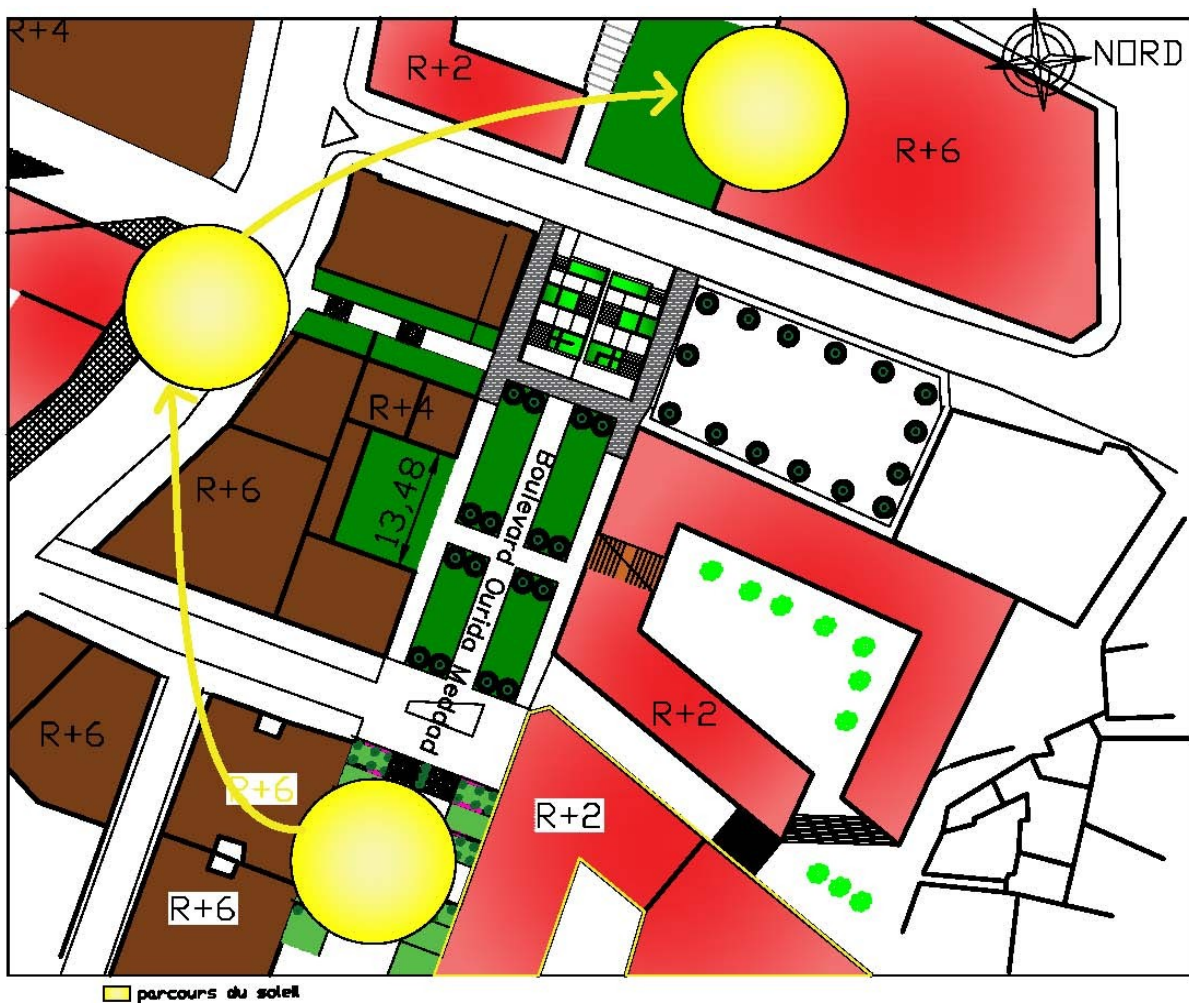
Figure 43. ensoleillement
