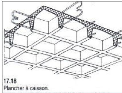
Figure 60.dalle à caisson
