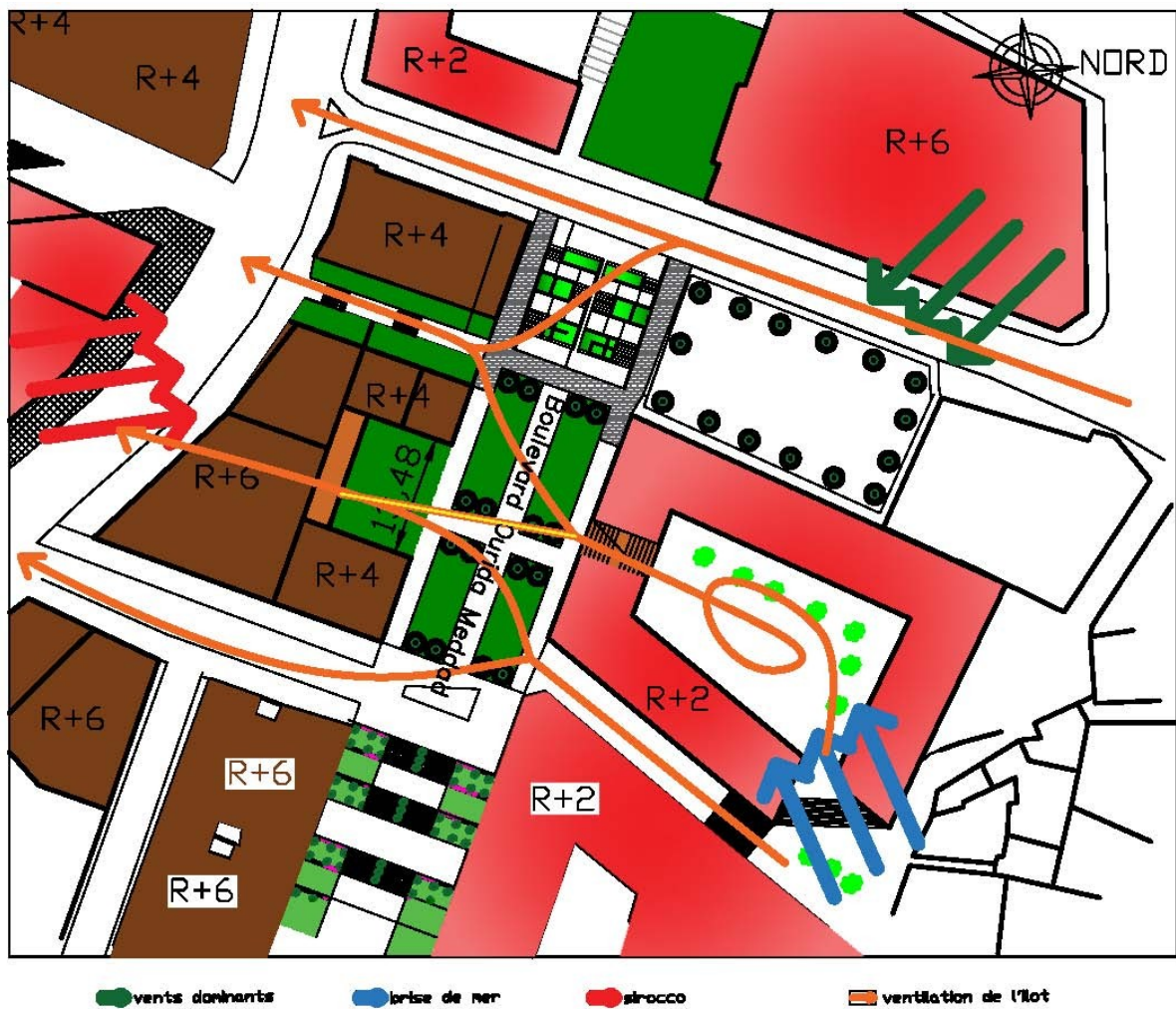
Figure 42.ventilation de l'ilot
