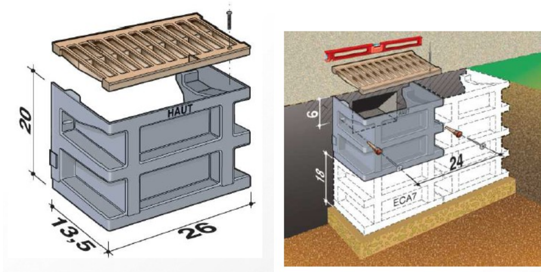
Figure 50.courette anglaise
