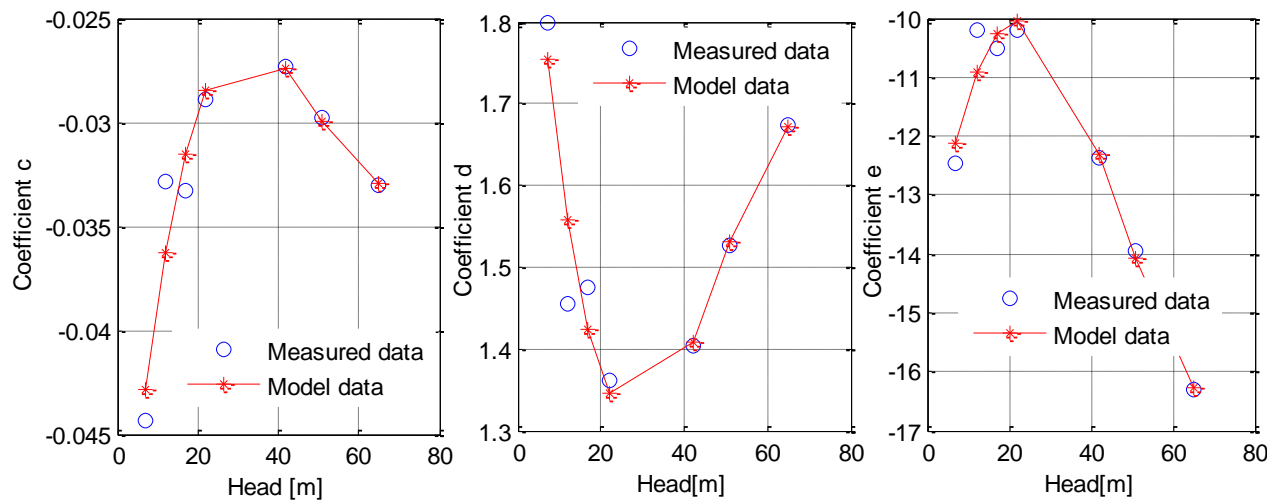
Figure 4.17 : Ajustement des coefficients de DP1.
