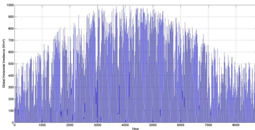
Figure 5.3: Irradiation Globale Horizontale d'une année du site de Ghardaia. La température d'un module PV dépend principalement de la température de l'air ambiante, de l'intensité de l'insolation et de la vitesse du vent.
