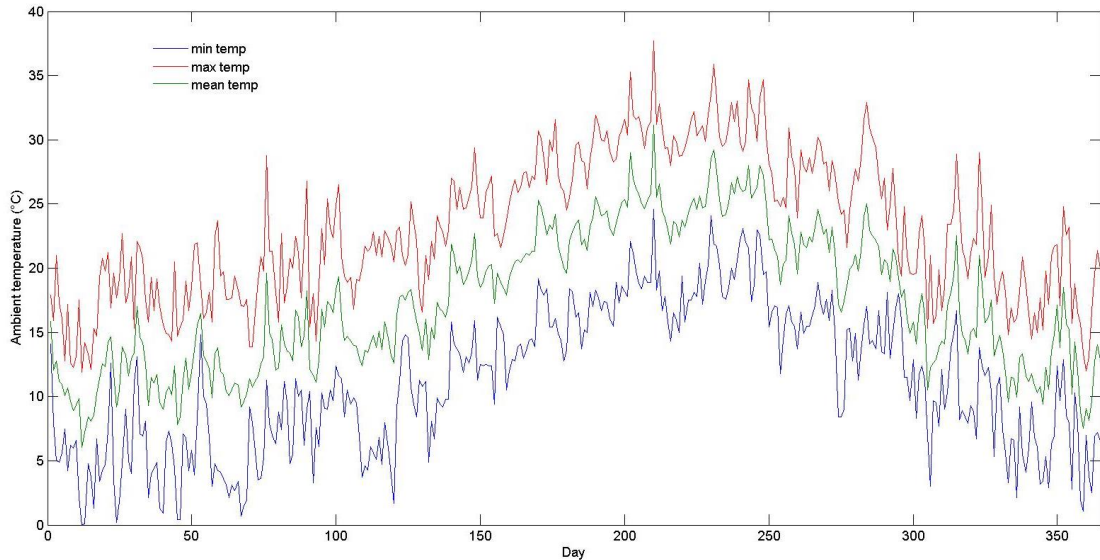
Figure 5.5 : Température ambiante horaire minimale, moyenne et maximale durant l'année du site de Ghardaia.
