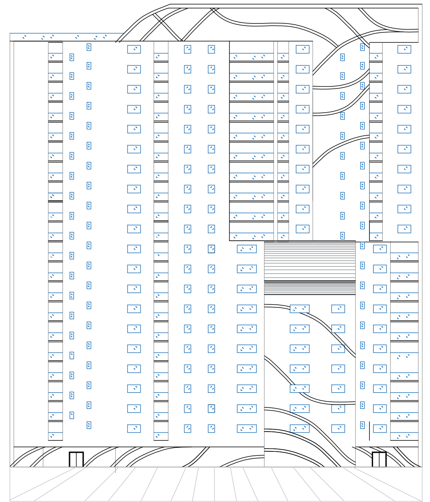
Façade Ouest
