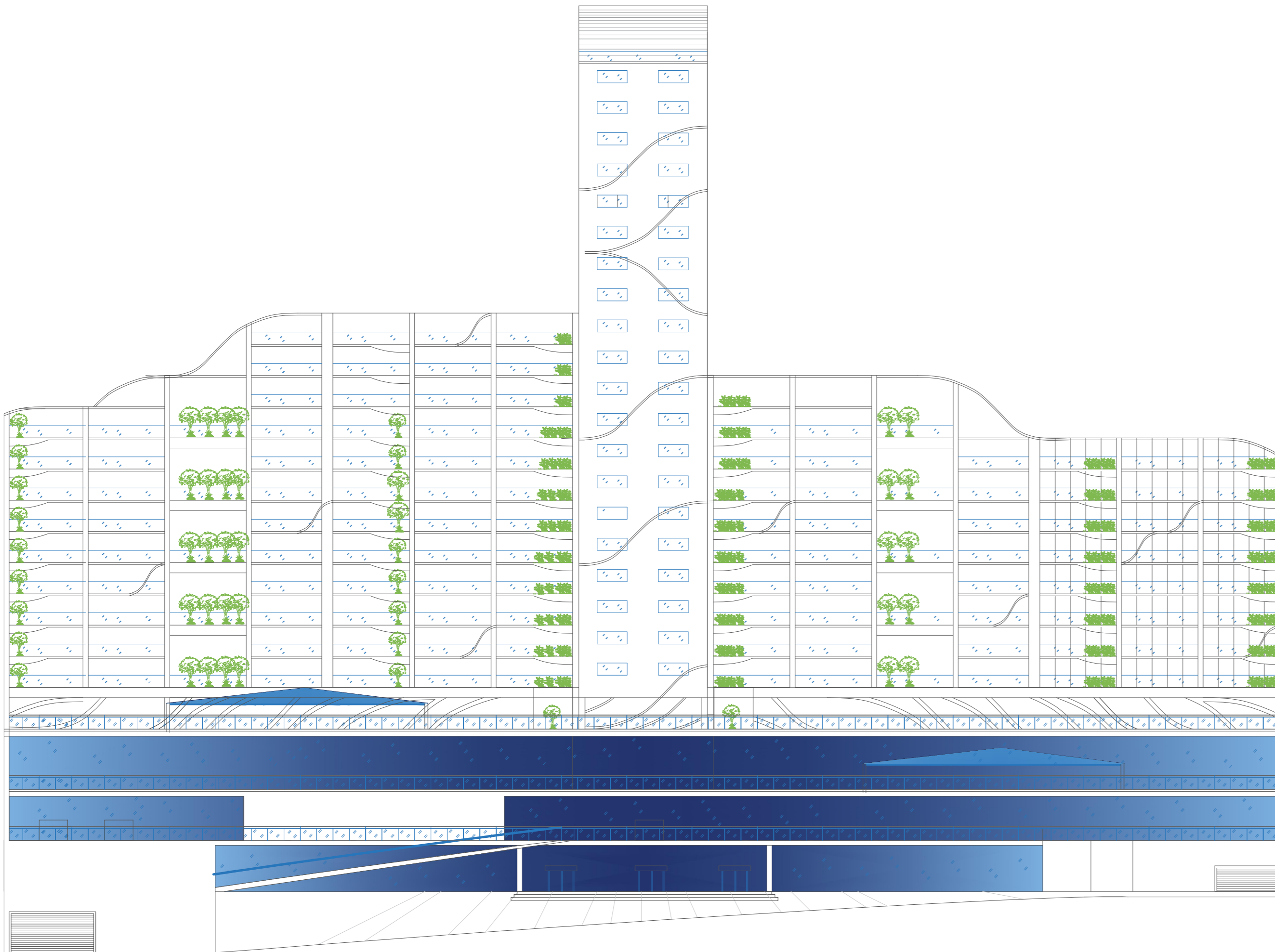
Façade Nord
