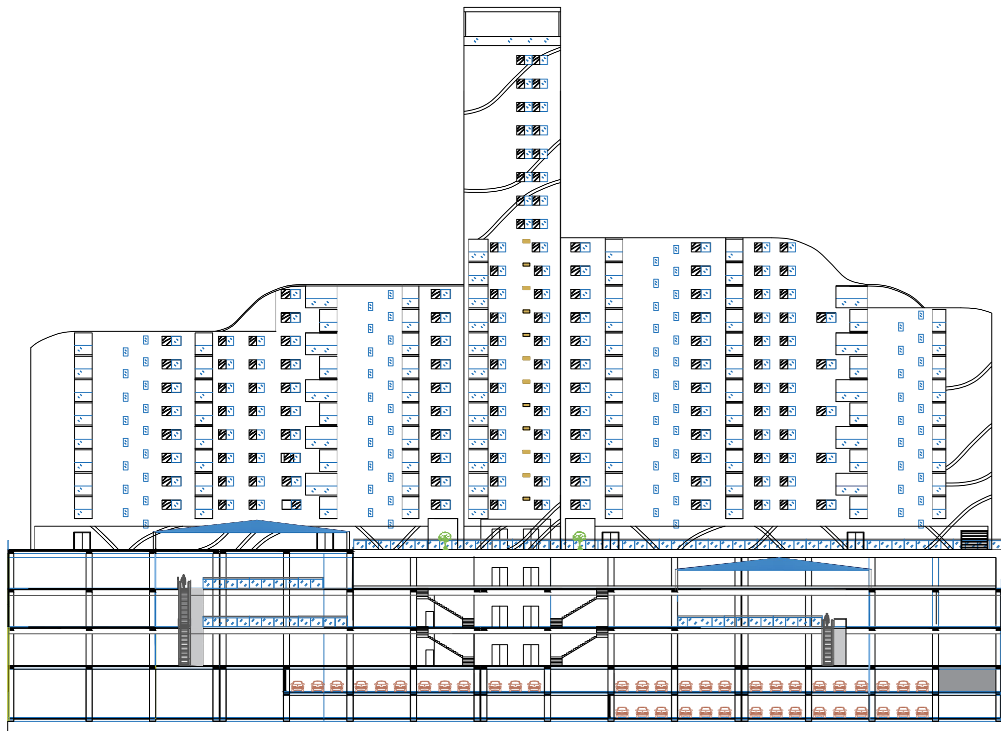
Coupe AA
