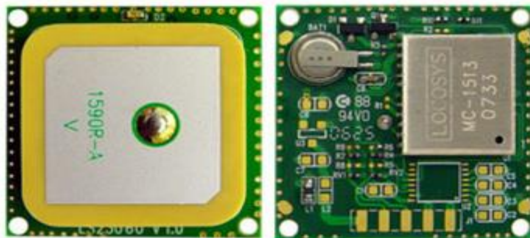
Figure.3.1 Faces avant et arrière du récepteur LS20031
