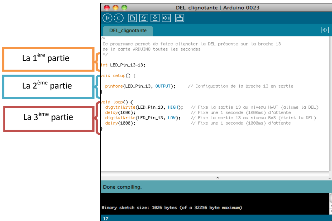
Figure.3.7 fenêtre graphique de l'EDI
