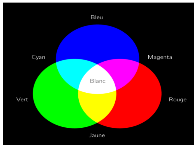
Figure 2-2 Synthèse additive des couleurs [50].
