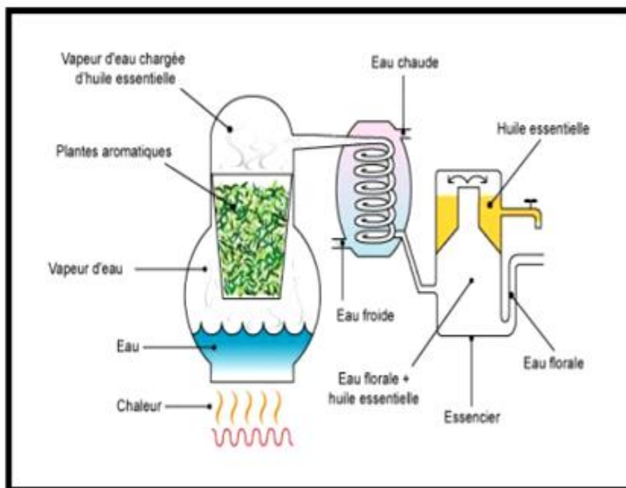
Figure. 17 : Schéma d'un montage d'entraînement à la vapeur d'eau (Bouaine, 2017).
