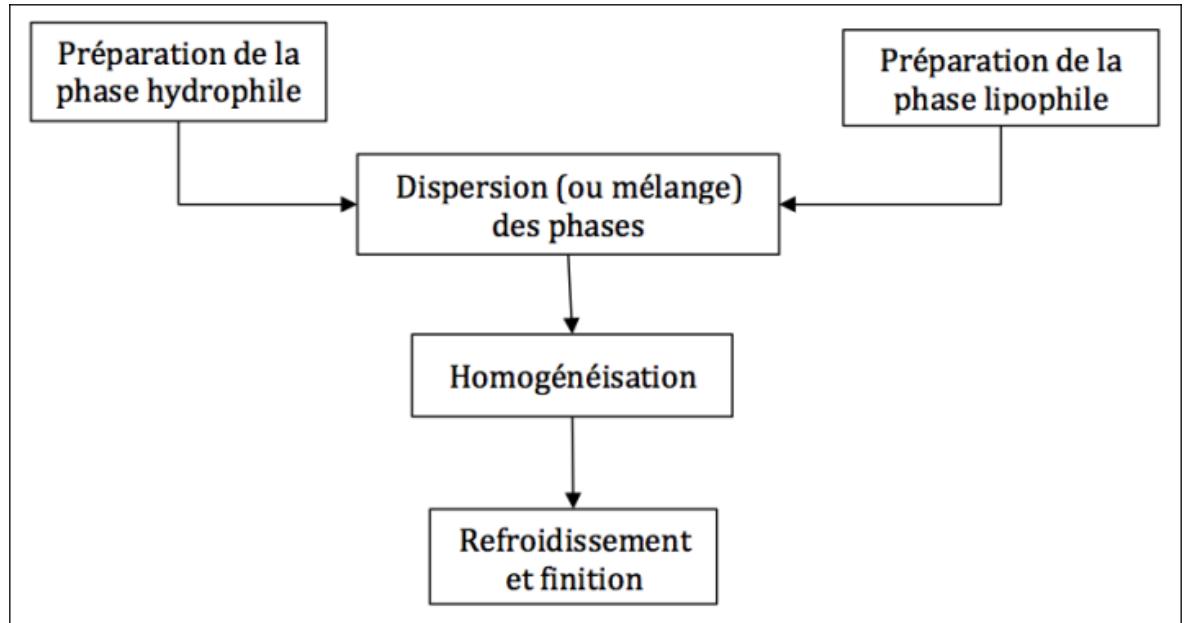
Figure 3.4 Diagramme du procédé de fabrication
