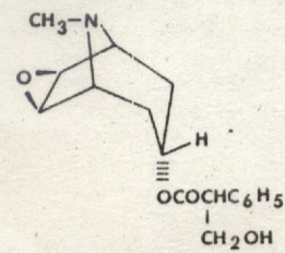
SCOPOLAMINE (d1) HYOSCYNE (1)
