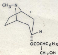
ATROPINE (d1) HYOSCYAMINE (1)
