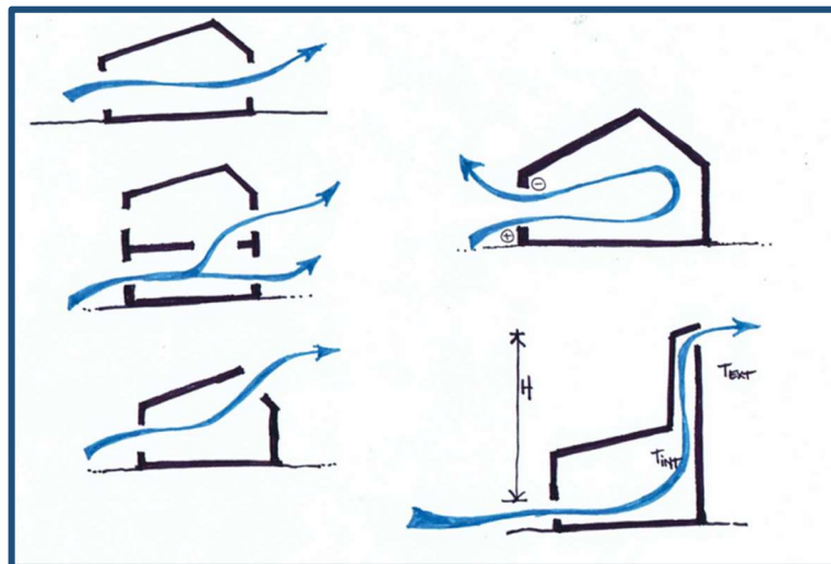
FIGURE.4.19 : Ventilation naturelle.
