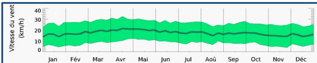
FIGURE.5.9 : Diagramme de la vitesse du vent en (Km/h) 0 Timimoune.
