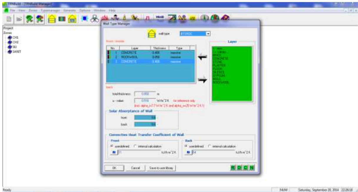
Figure IV.18. définition des murs extérieurs de la maison
