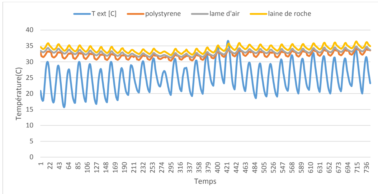
Figure V.4. Evolution de la température intérieure de la maison pendant le mois d'Aout
