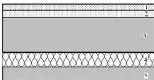
Figure III.5. Plancher bas sur terre-plein
