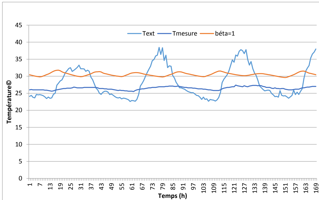
Figure V.8. Evolution de la température intérieure de la maison pendant une semaine d'Aout (2013)
