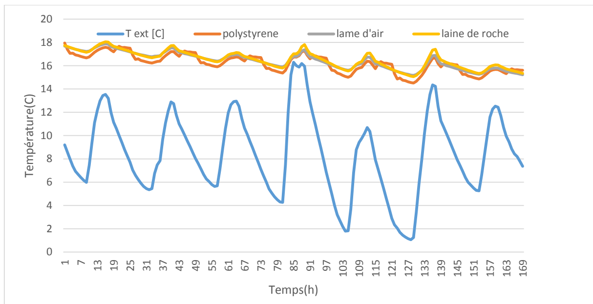
Figure V.3. Evolution de la température pendant une semaine de Janvier (du 07au14)
