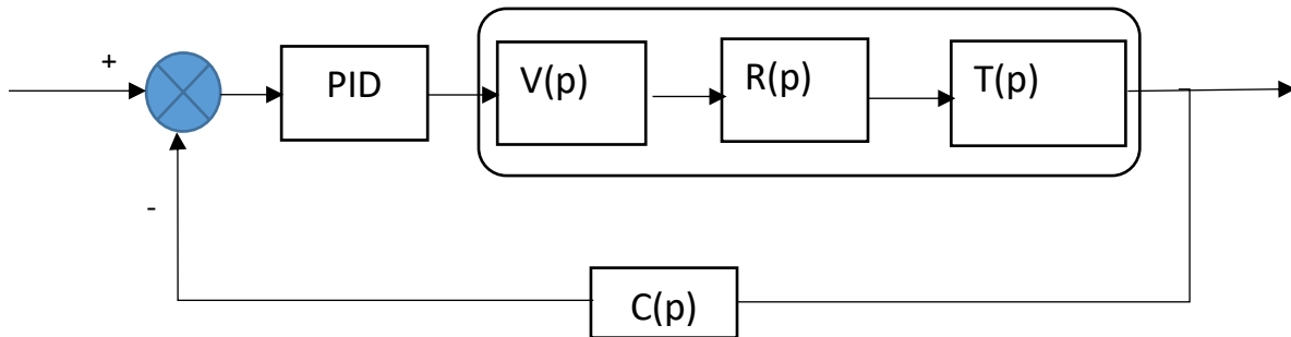
Figure III.4 : le schéma de la boucle de régulation.
