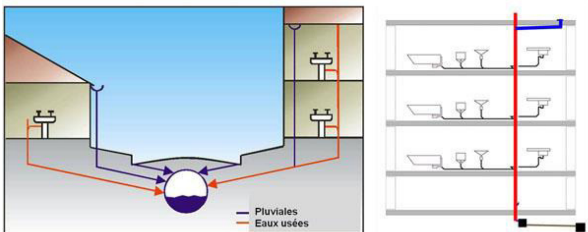
Figure III.1 : système unitaire
