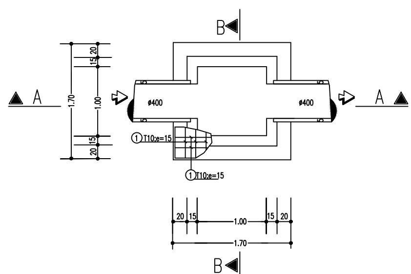
FERRAILLAGE RADIER
