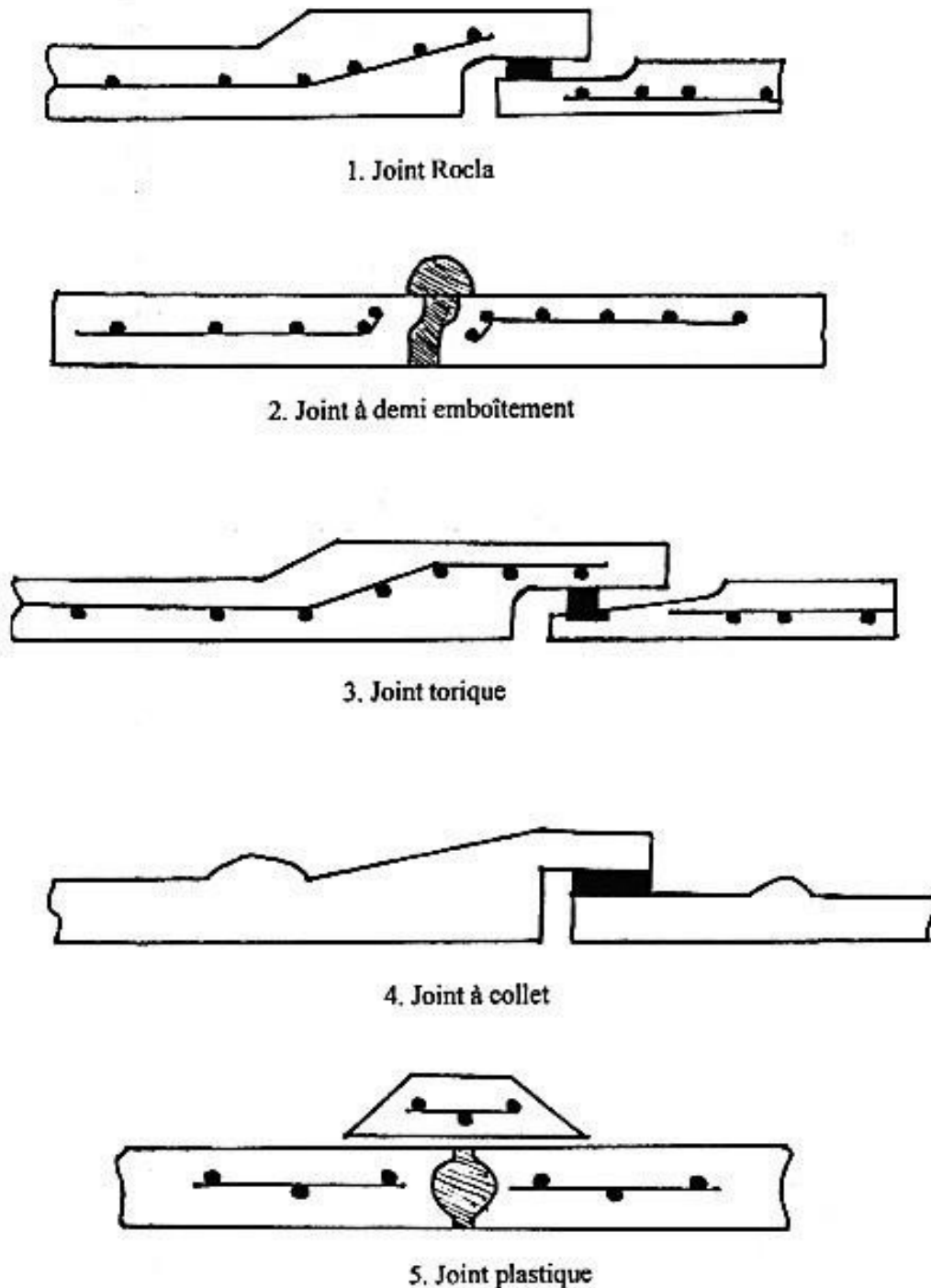
Figure V.2 : Divers joints sur tuyau en béton
