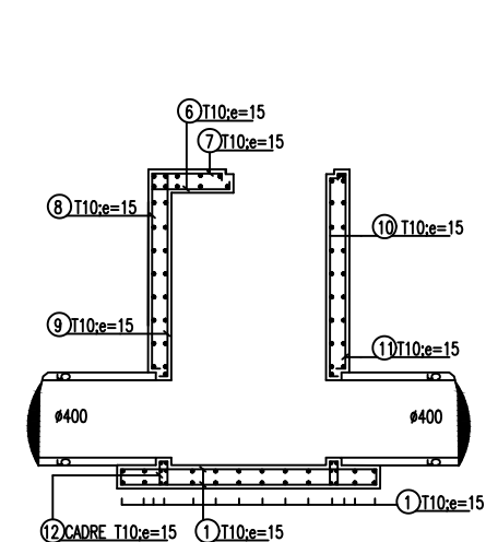
FERRAILLAGE COUPE A-A
