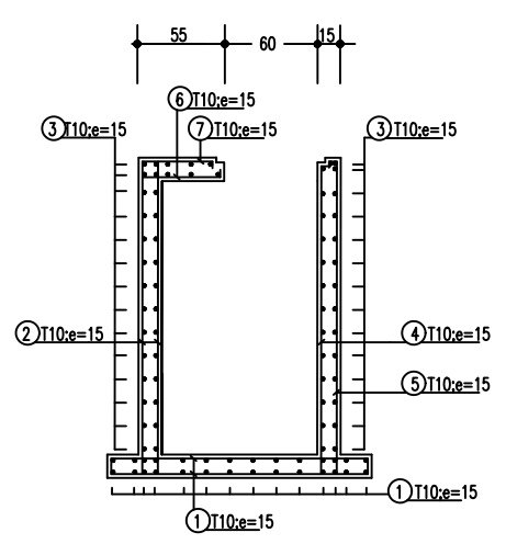
FERRAILLAGE COUPE B-B
