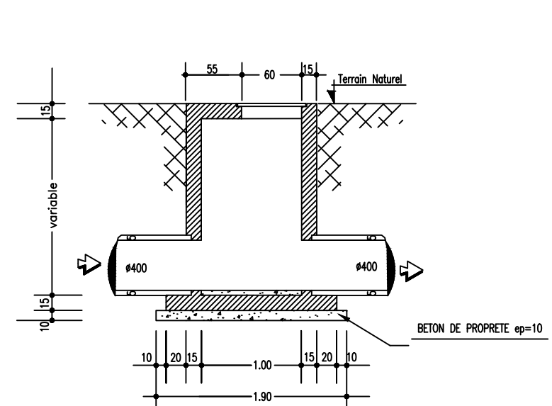
- COUPE A-A -
