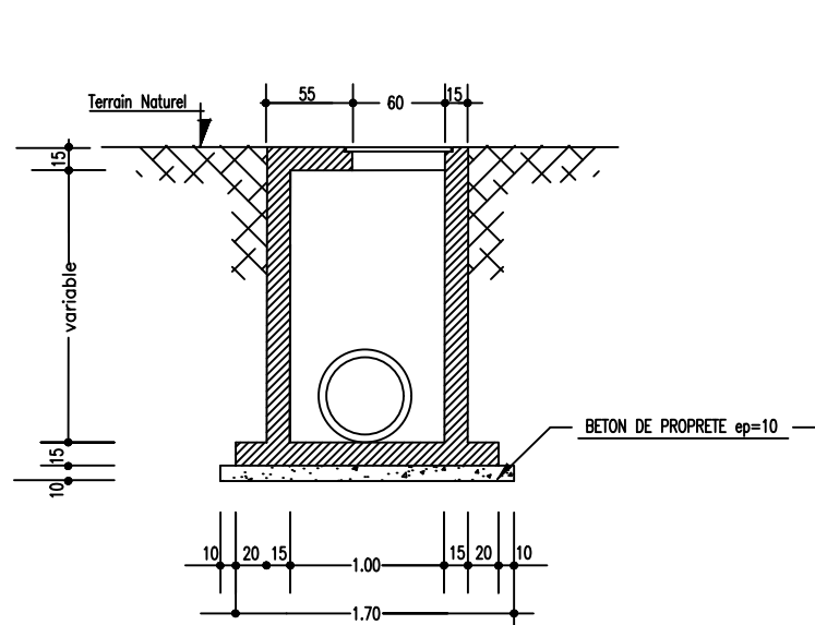
- COUPE B-B -
