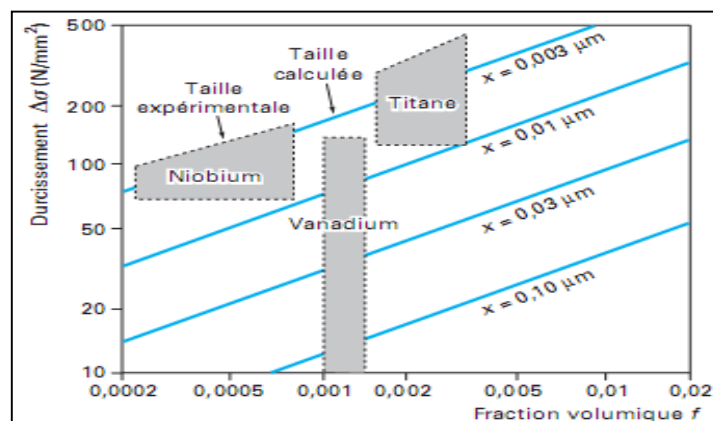
Figure I.2 : Durcissement en fonction de la taille et de la quantité des précipités [6]
