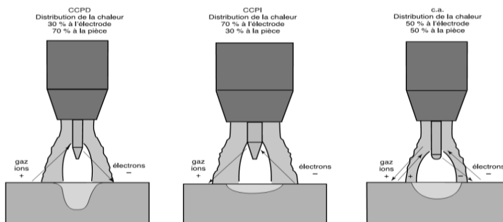
Figure II.3 : Distribution approximative de la chaleur lors du soudage TIG selon les polarités CCPD, CCPI et C.A
