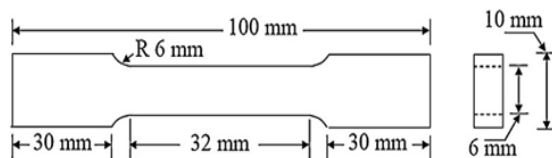
Figure III.14 : L'éprouvette de traction la norme ASTM (E8/E8M – 09) [33]
