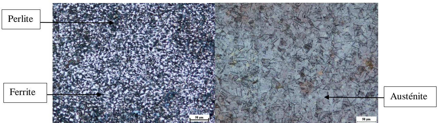
Figure IV.2 : Micrographies les matériaux de base : X70 (à gauche) et 304L
