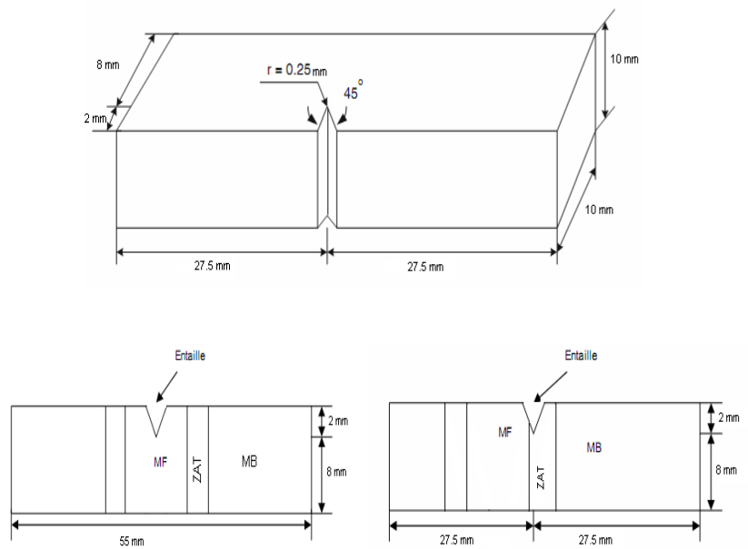
Figure III. 9 : Forme de l'éprouvette de résilience et la position de l'entaille.
