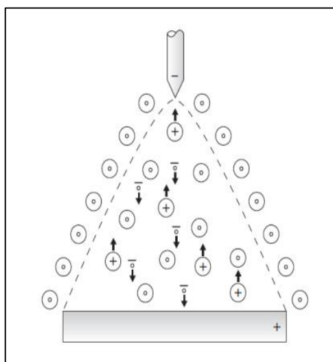
Figure II.2 : Principe d'un arc électrique [21]
