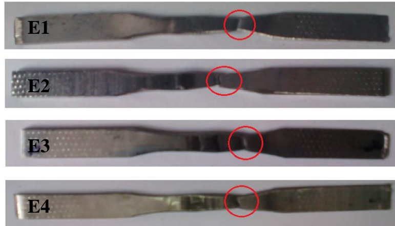
Figure.IV.8 : les éprouvettes après de tractions
