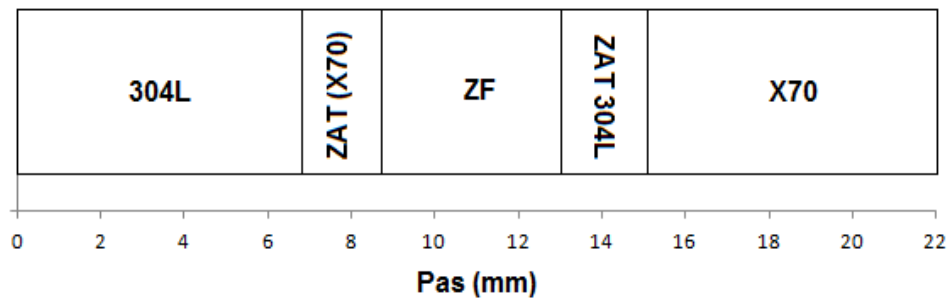
Figure IV.4: Montrant l'axe X des profils de microdureté
