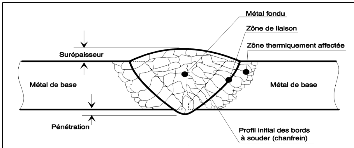
Figure II.4 : Structure d'une soudure [26]
