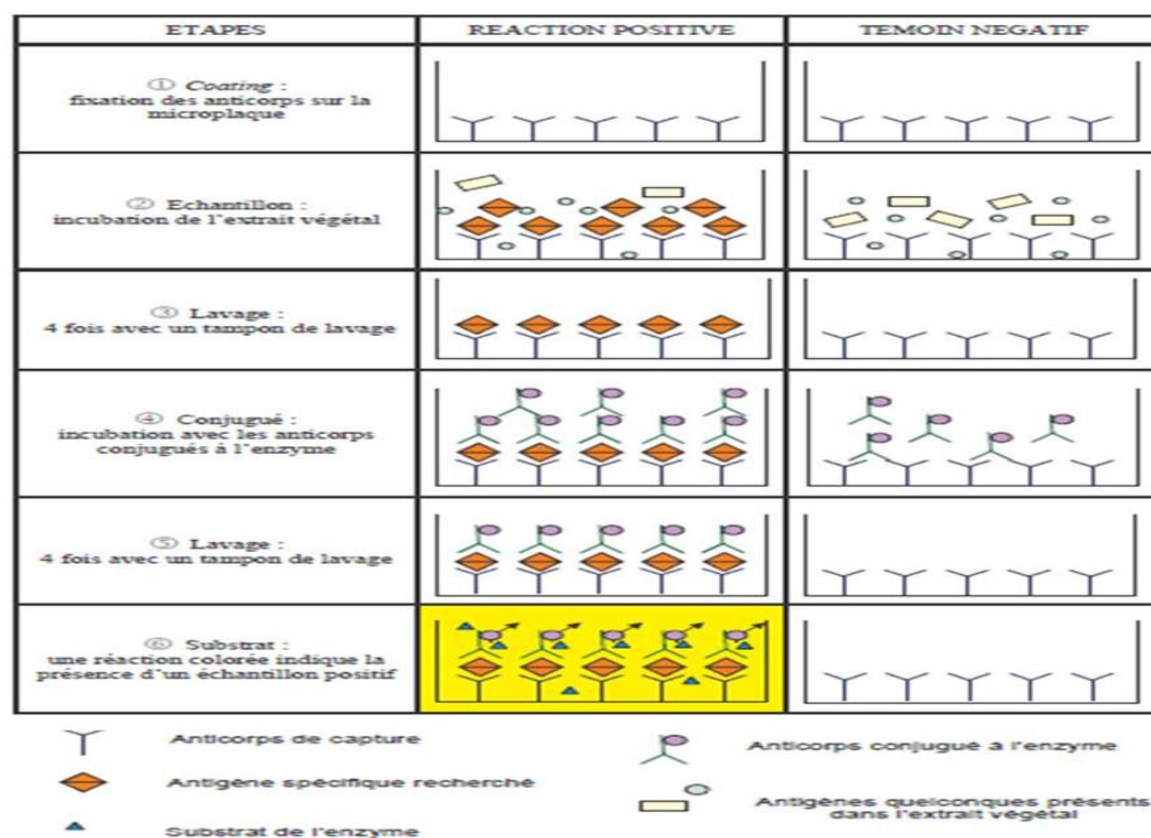
Figure 9: Schématisation du principe de la technique ELISA
