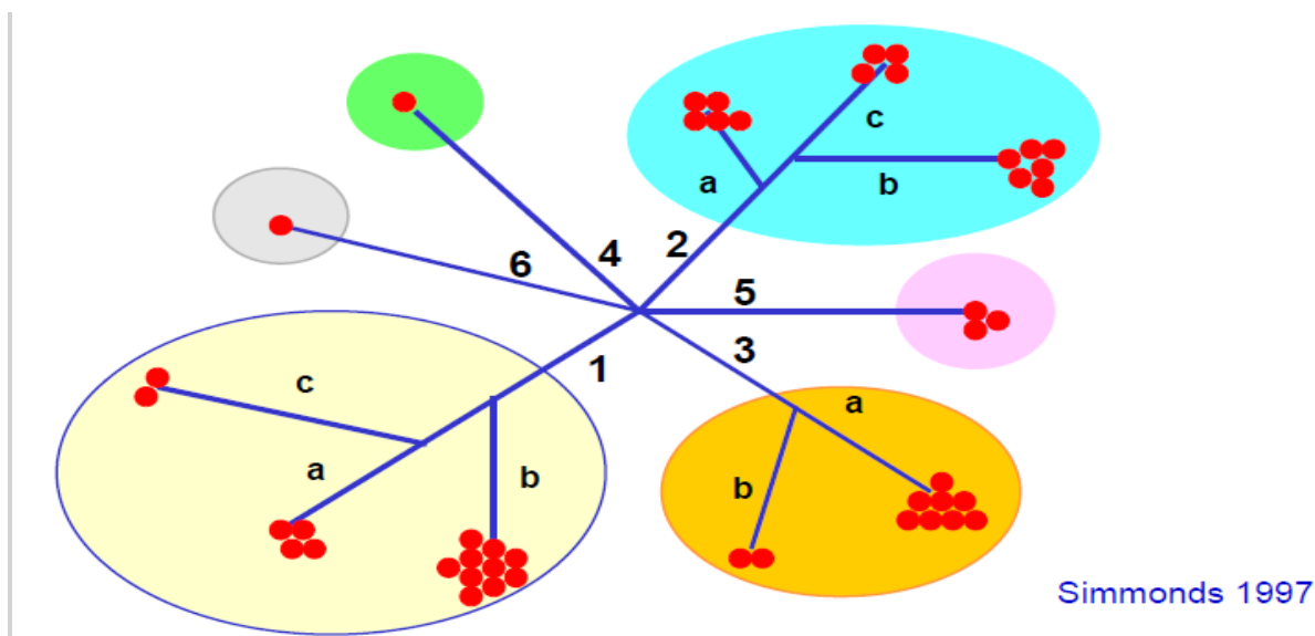
Figure 4: Schématisation des différents génotypes et sous types du VHC sous forme d'un arbre phylogénétique (10)
