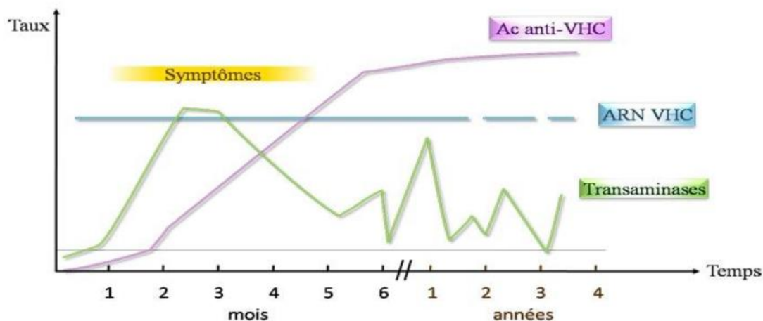
Figure 8: Evolution des marqueurs sérologiques au cours d'une hépatite C chronique
