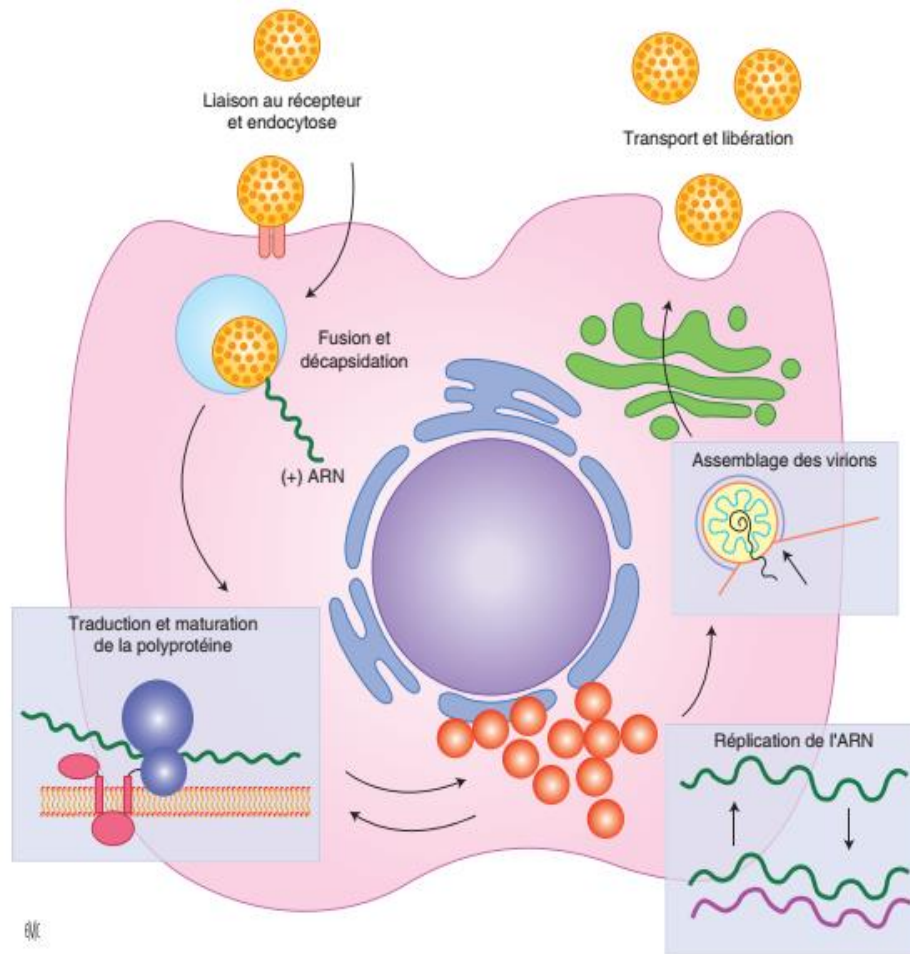
Figure 3 Schématisation du cycle de multiplication du VHC (80)
