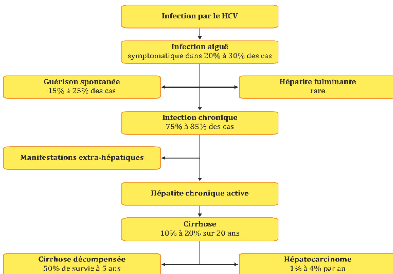
Figure 5: Histoire naturel de l'infection par le VHC
