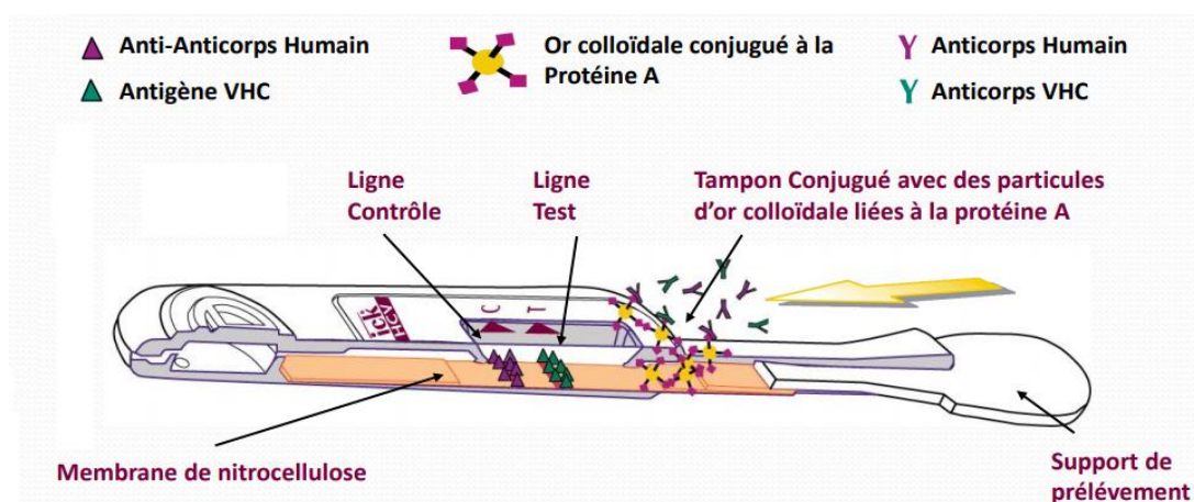
Figure 10: Schématisation du fonctionnement de l'oraquick
