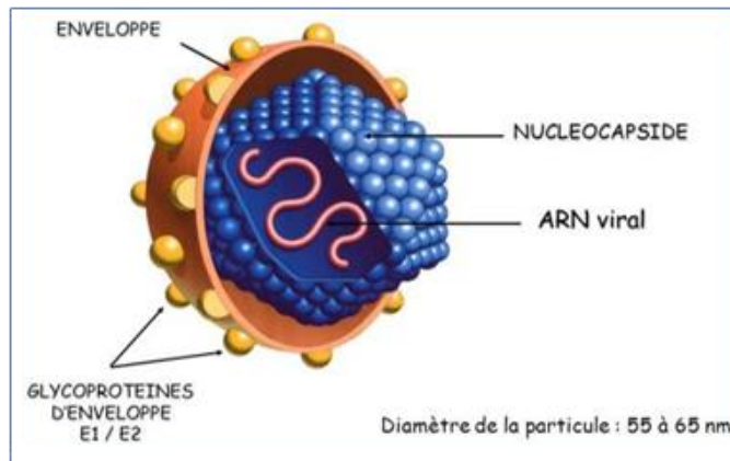
Figure 1: Représentation schématique de la particule virale du VHC
