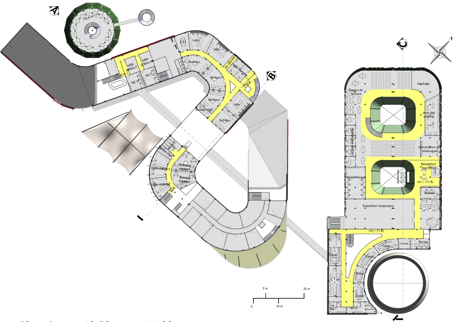
Plan niveau +10.00 m et + 11.00 m
