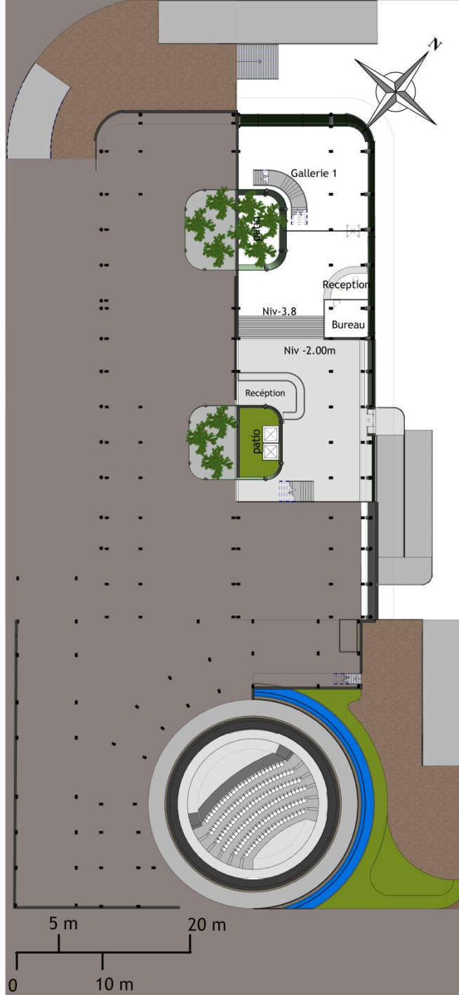
Plan niveau -2.00 m
