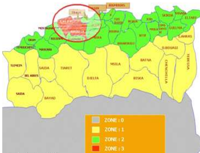
Figure37-carte de zonage sismique de nord algérien. (Source : Google image)
