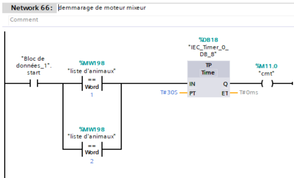
Figure III.9 : Démarrage du moteur mixeur
