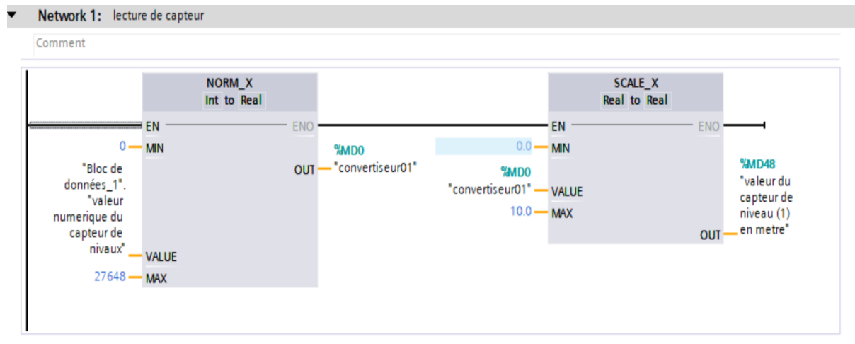
Figure III.5 : Traitement de l'information mesure par le capteur
