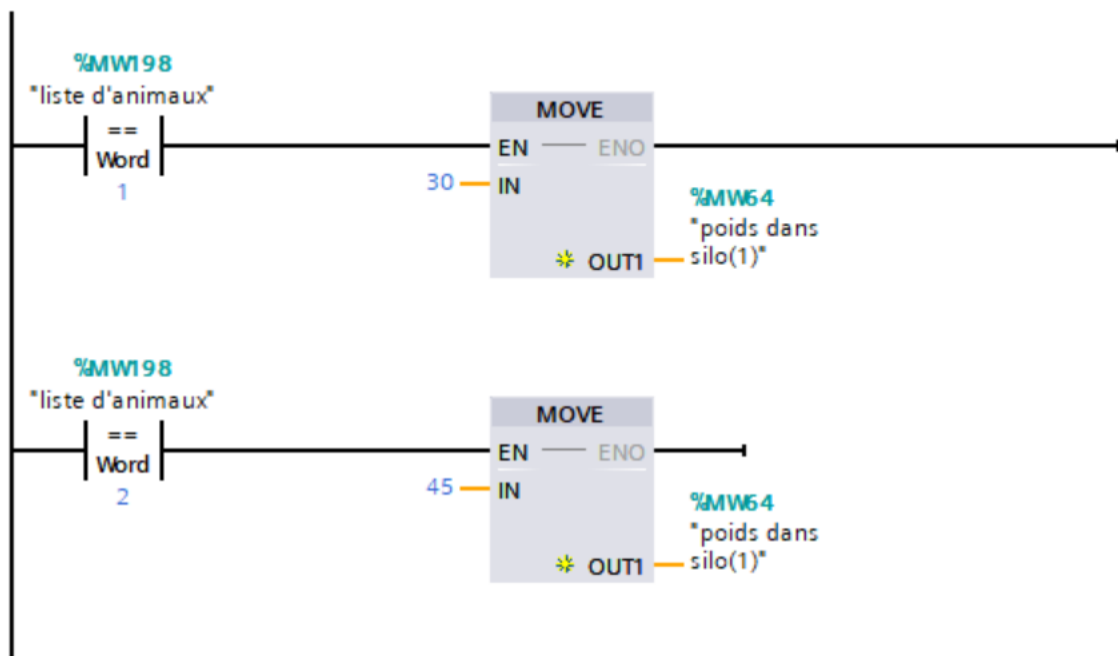
Figure III.6 : Réseau pour choisir le type d'animal
