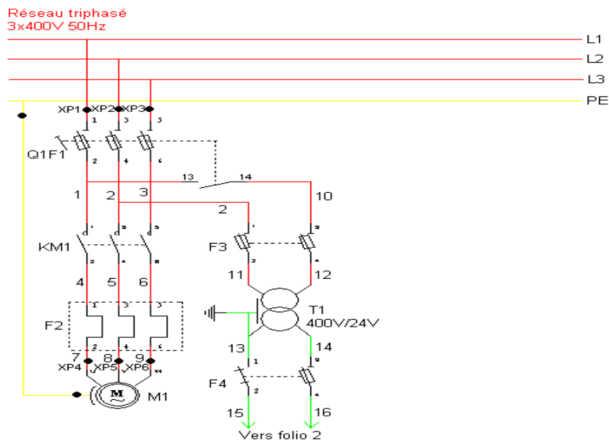
Figure II.19 : Partie puissante d'un schéma électrique
