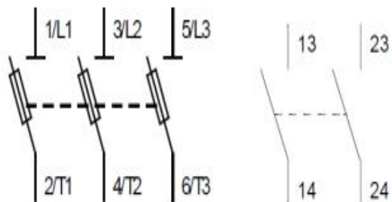
Symboles : en circuit de puissance et en circuit de commande
