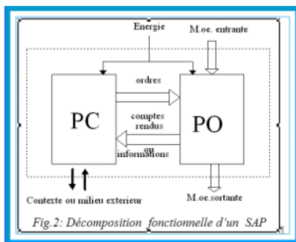
Figure II.1 : Structure d'un système automatisé
