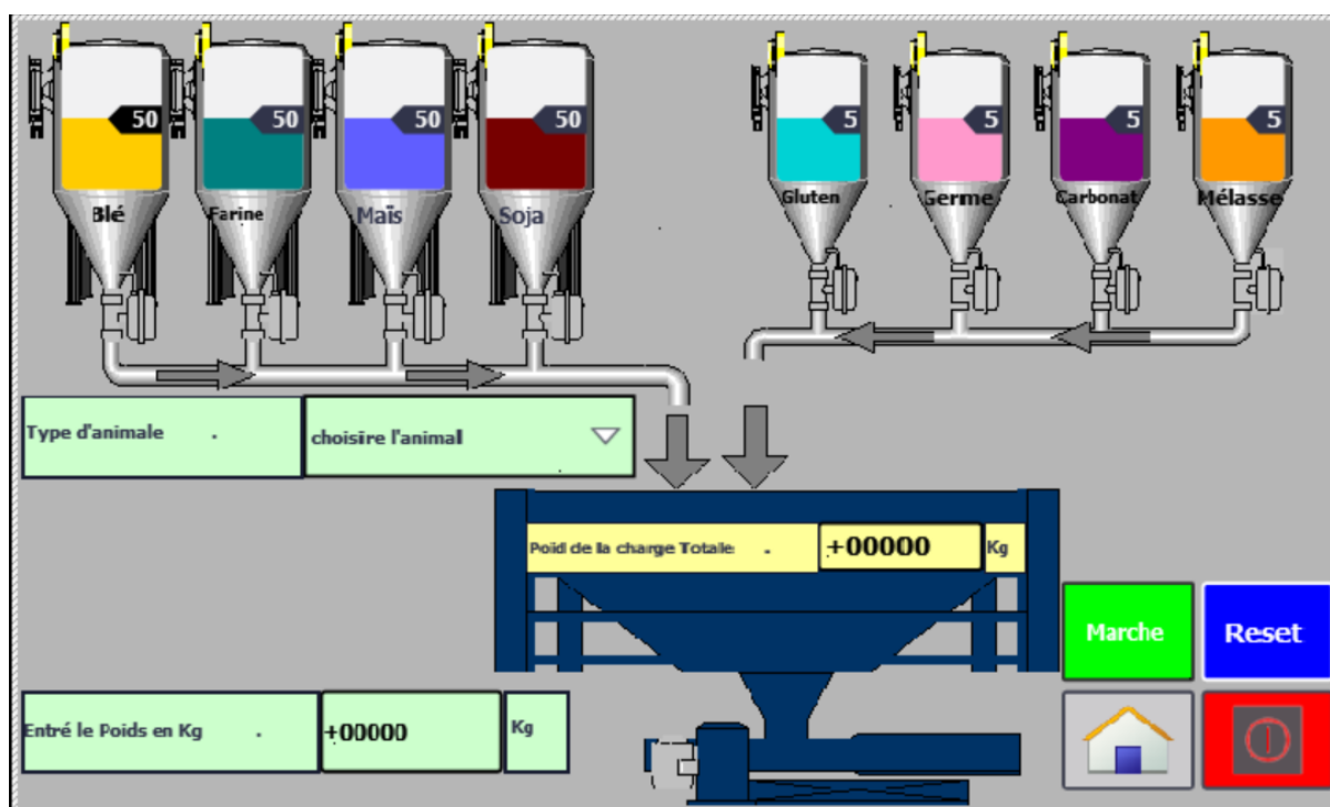
Figure III.15 : Vue de notre system
