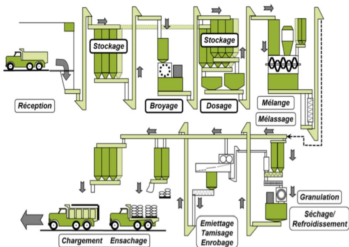
Figure I.5 : Processus de fabrication d'aliment.
