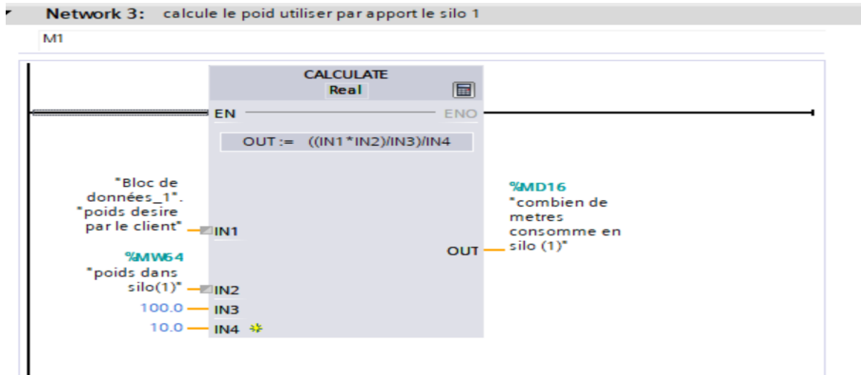
Figure III.7 : Calcul de la quantité du produit nécessaire dans silo 1.
