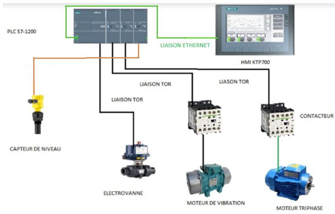
Figure III.1: Schéma de câblage de notre système
