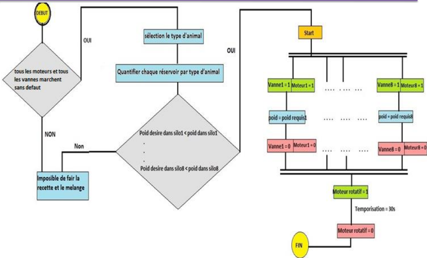
Figure III.2 : L'organigramme de fonctionnement.
