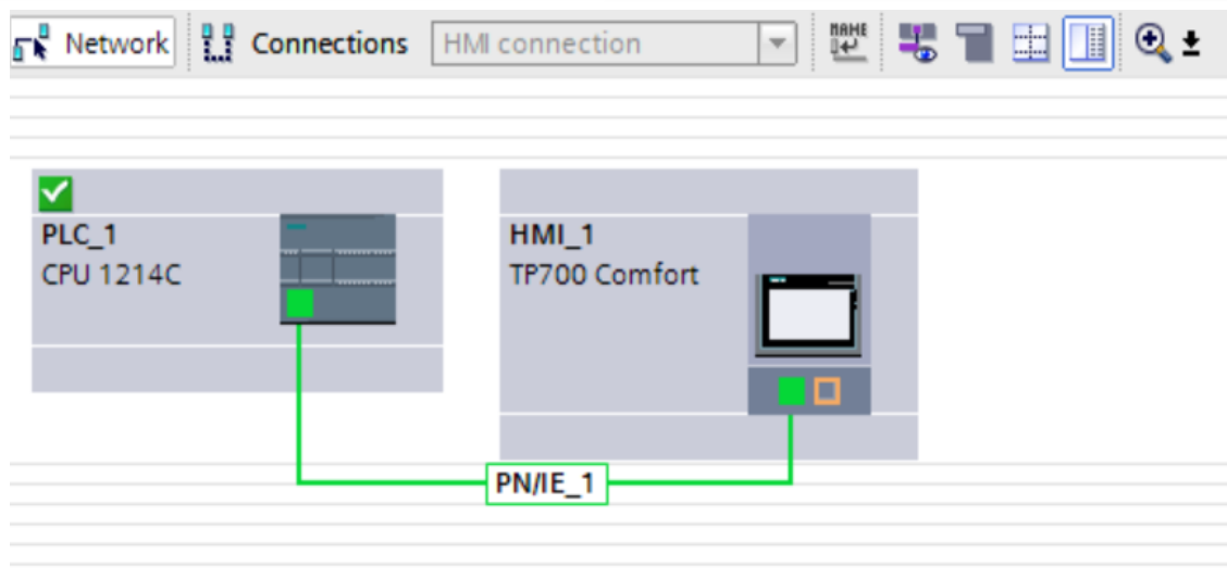
Figure III.10 : Configuration de la liaison Automate-IHM
