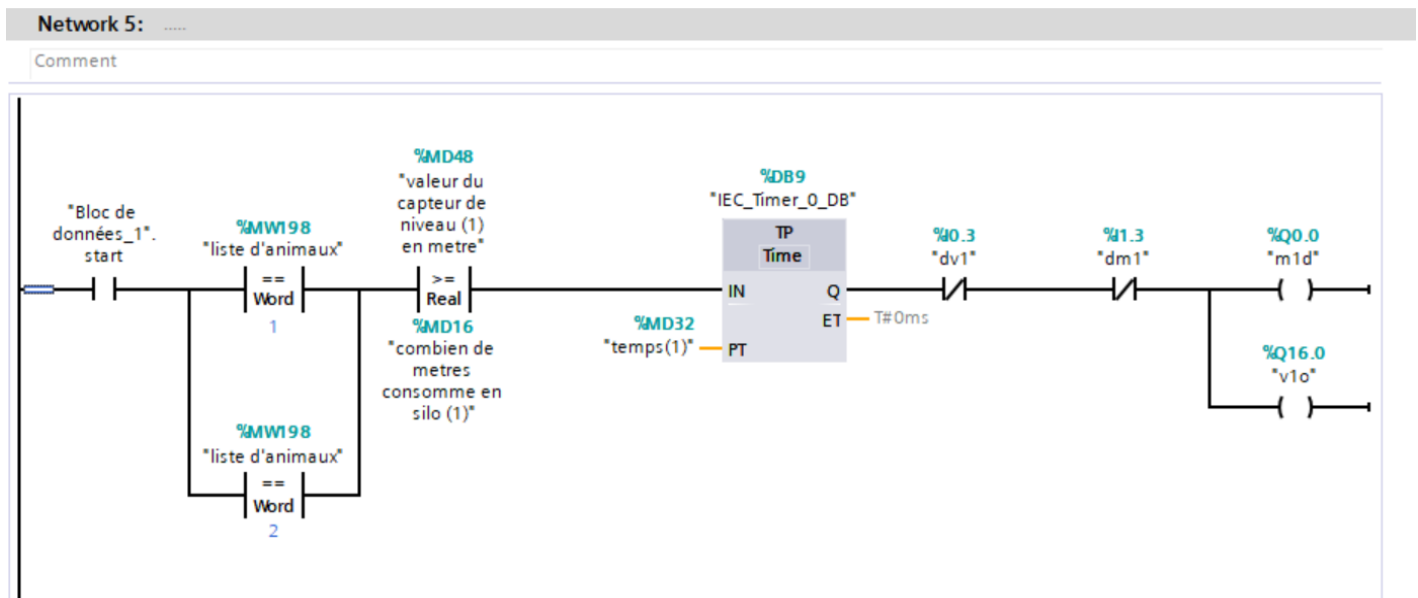
Figure III.8 : Démarrage du moteur vibrant 1 et l'ouverture de la vanne 1
