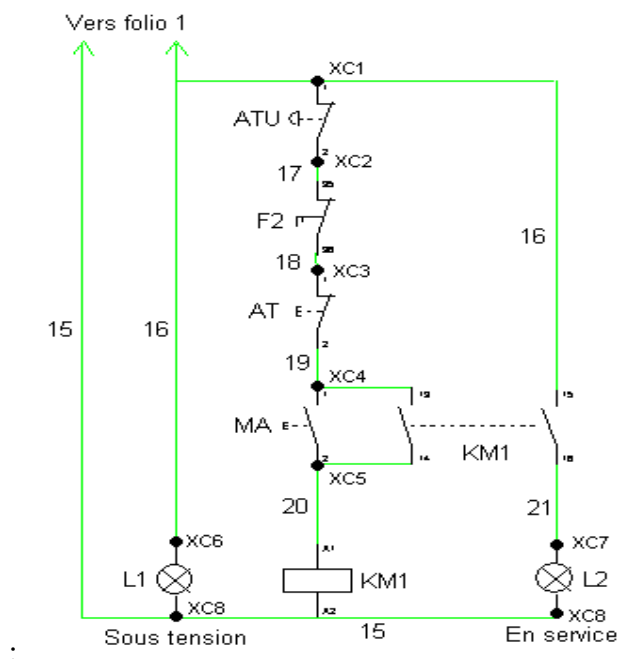
Figure II.18 : Partie commande d'un schéma électrique
