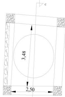
Vue en plan C1 ech:1/50
