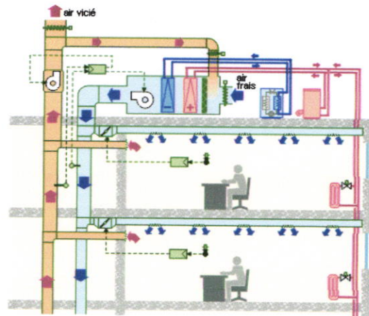
Figure n°=24 Exemple de climatisation centrale
