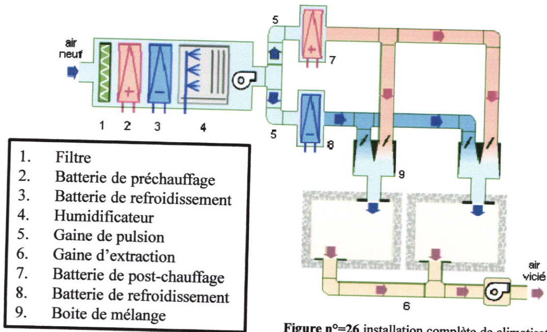
Figure n°=26 installation complète de climatisation
