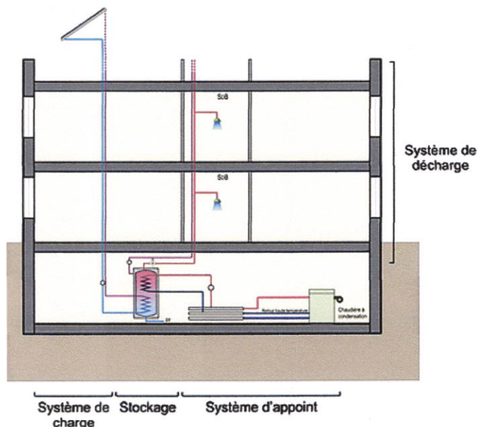
Figure n°=30 Le système de stockage
