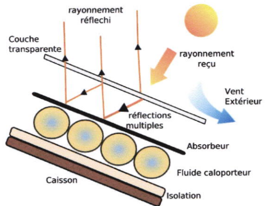
Figure n°=29 les composants d'un capteur solaire
