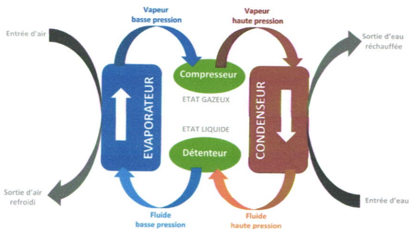
Figure n°=25 Principe de la pompe à chaleur
