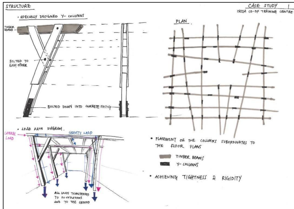
Figure 16 . représente la structure des piliers en Y. source : https://estelleang.wordpress.com/2015/07/08/cassia-co-op-training-centre/
