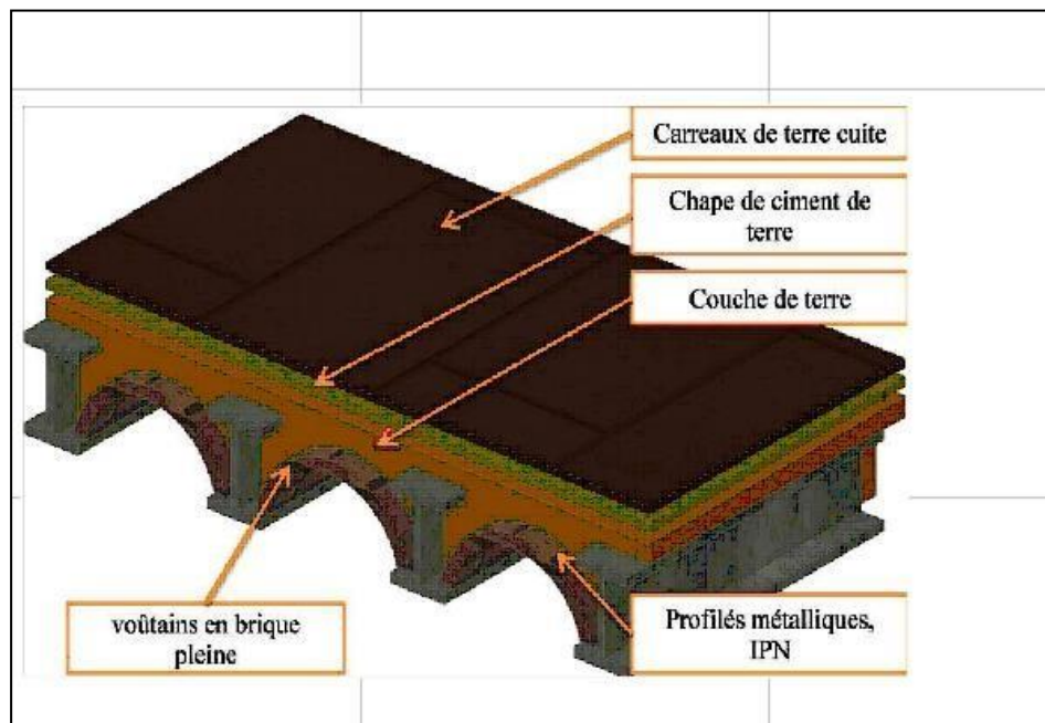
Figure 50 détail du plancher en voutains
