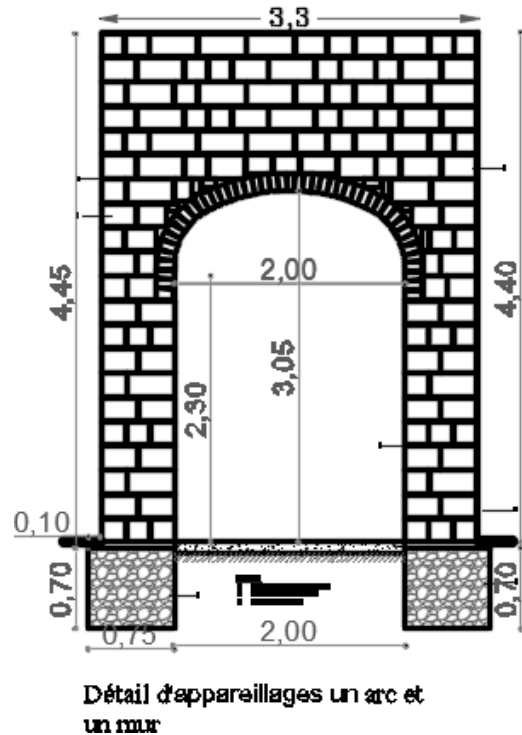
Figure 57 détail d'appareillage d'un arc avec un mur
