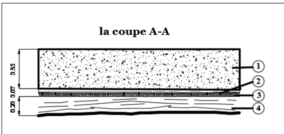
Figure 52 coupe sur le plancher traditionnel
