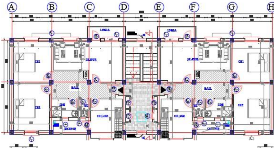
Figure 22. Plan 1 er étage du logement du centre.
