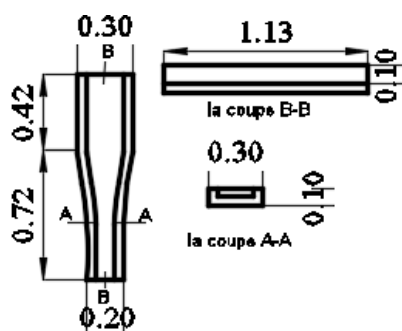
Détail des gargouilles en terre cuite
