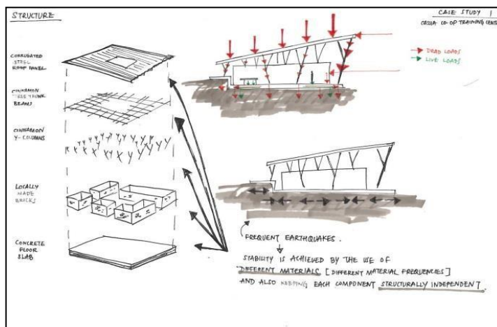
Figure 15. la structure générale du centre. Source :
