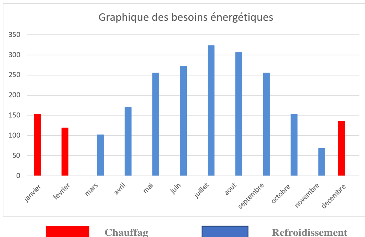
Figure 60 : graphique des besoins énergétiques d'une construction en brique creuse
