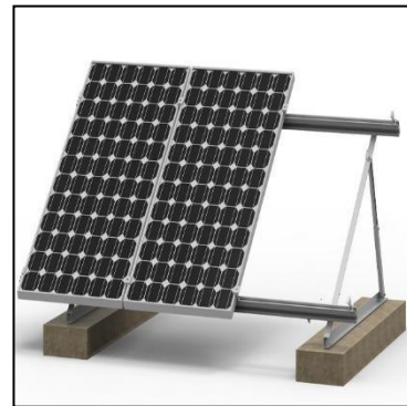
Figure 66 Le montage des panneaux solaire
