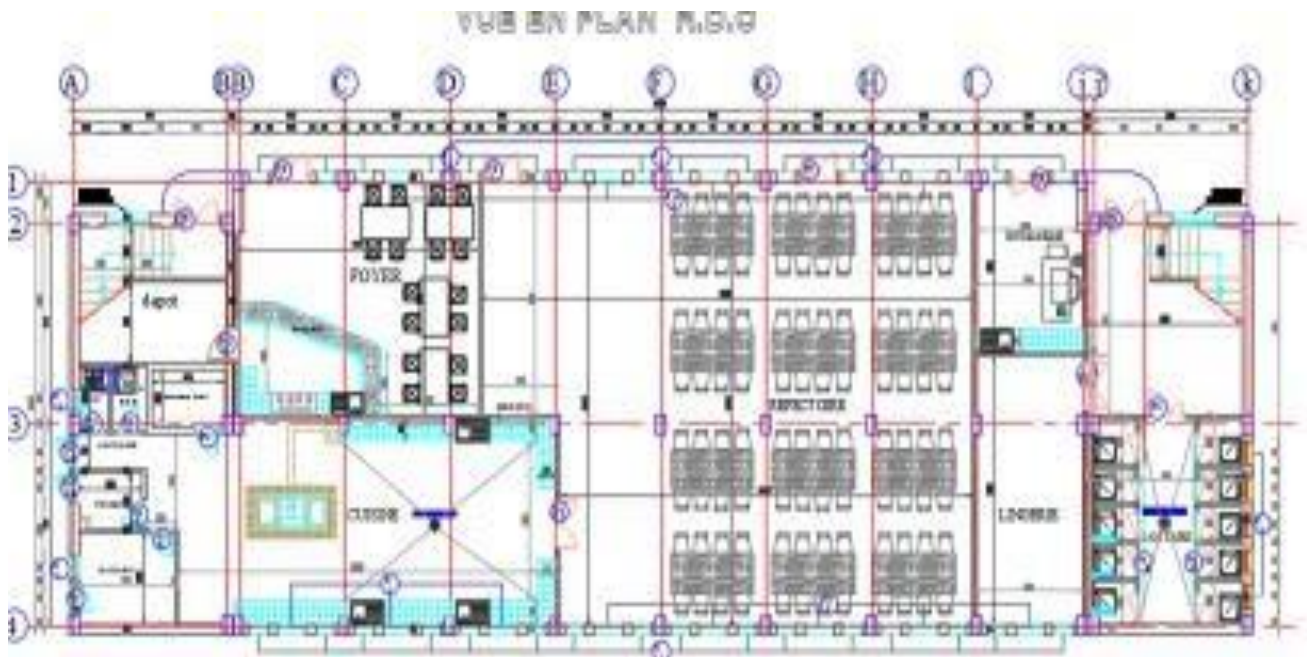
Figure 24 plan RDC des salles de cours + sanitaire.
