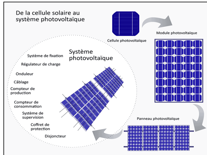
Figure 64 les composants de système PV (une cellule, un module, un panneau PV)
