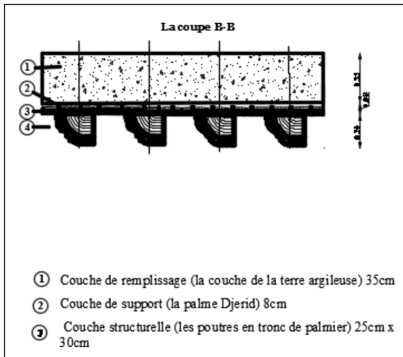
Figure 51 détail du plancher traditionnel
