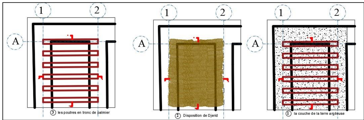
Figure 53 les différentes couches du plancher traditionnel
