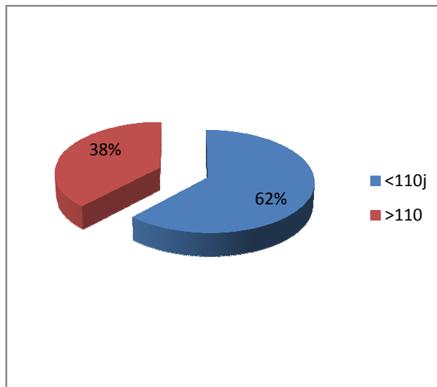
Figure 14 : Intervalle vêlage-IF.
