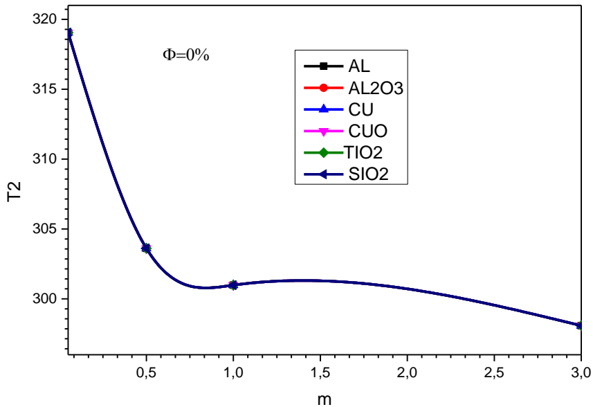
Figure IV.100: Variation du température T2 (eau/nanofluides) en fonction de débit massique pour la concentration \Phi=0\%
