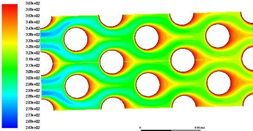
Figure IV.54: contour de température concentration \phi=3\% et débit massique m=0.05\text{kg/s} ( \text{TiO}_2 )
