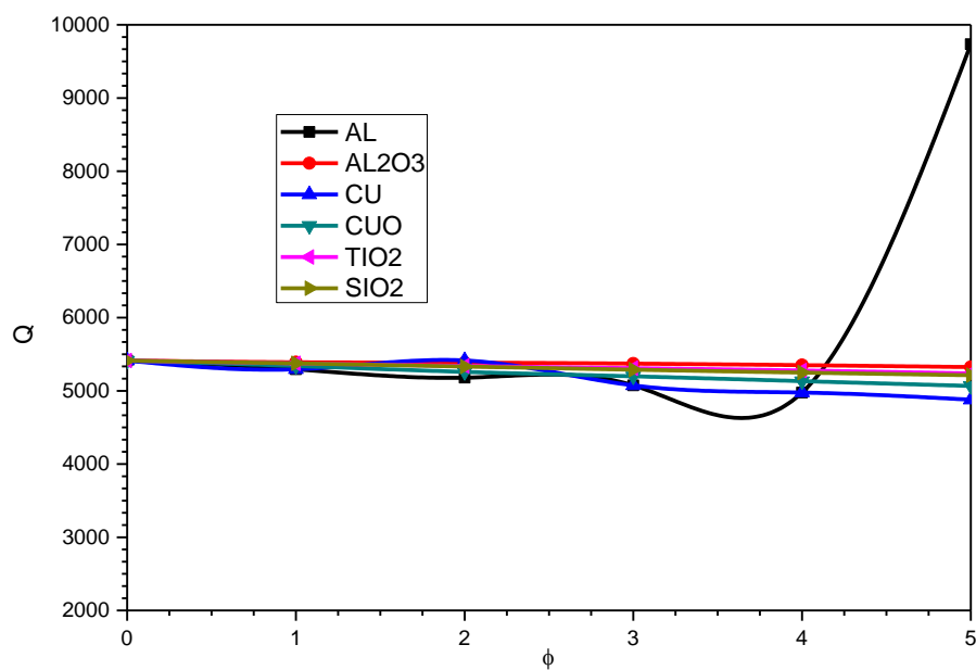
Figure IV.95: Variation du flux de chaleur Q (eau/nanofluides) en fonction de la concentration \Phi pour débit massique m=0.05 Kg/S
