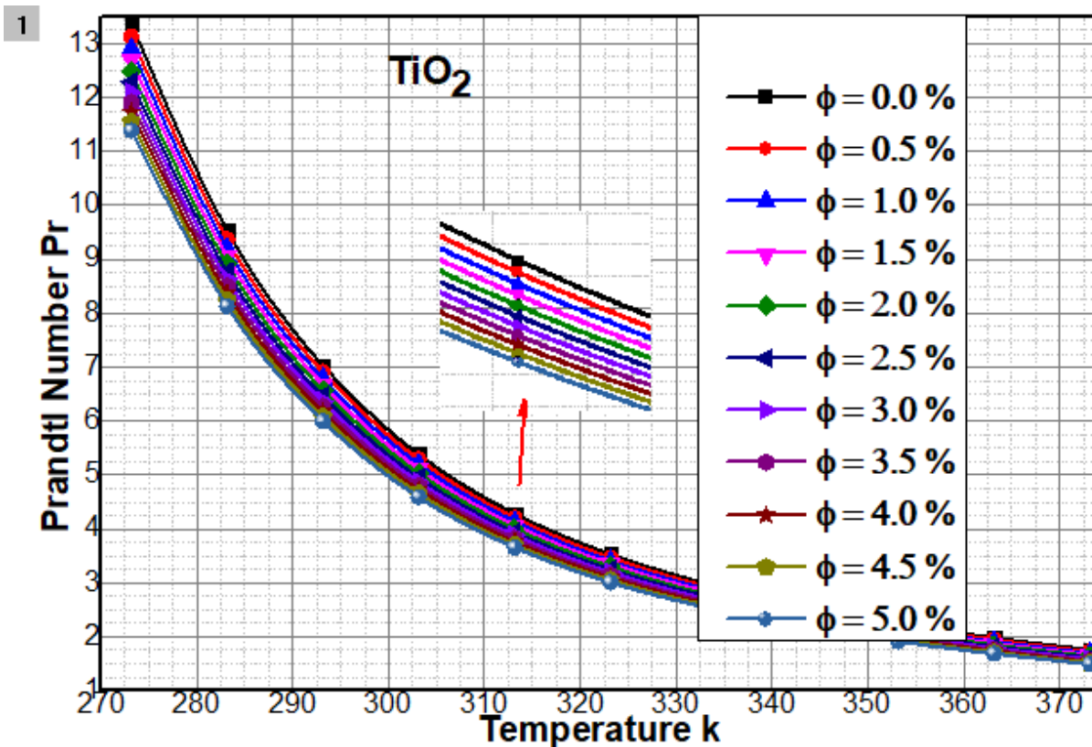
Figure III.21 : Évolution du nombre Pr en fonction de la température pour une concentration de NP différente
