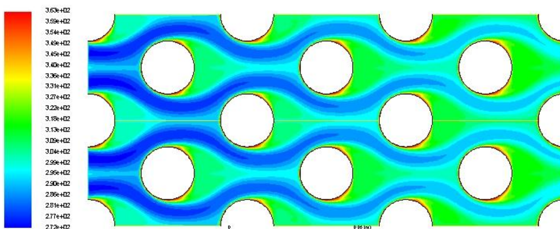
Figure IV.63: contour de température concentration \emptyset=5\% et débit massique m=0.5\text{kg/s} ( \text{CuO} )
