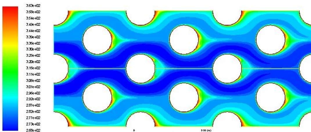
Figure IV.57: contour de température concentration \phi=4\% et débit massique m=3\text{kg/s} (CuO)
