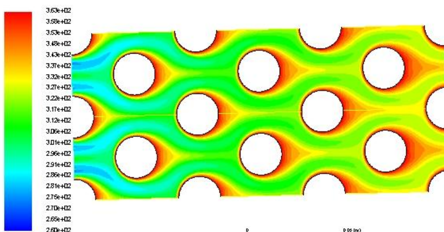
Figure IV.58: contour de température concentration \phi=4\% et débit massique m=0.05\text{kg/s} (TiO 2 )
