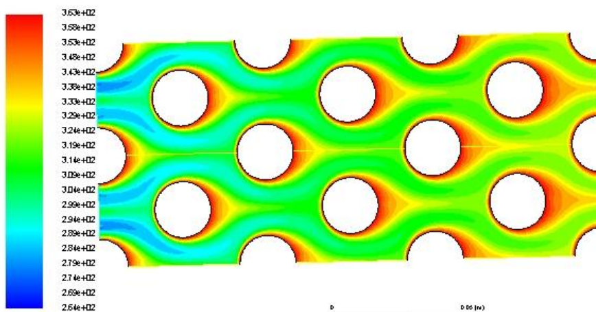
Figure IV.50: contour de température pour concentration \text{Ø}=2\% et débit massique m=0.05\text{kg/s} (AL 2 O 3 )
