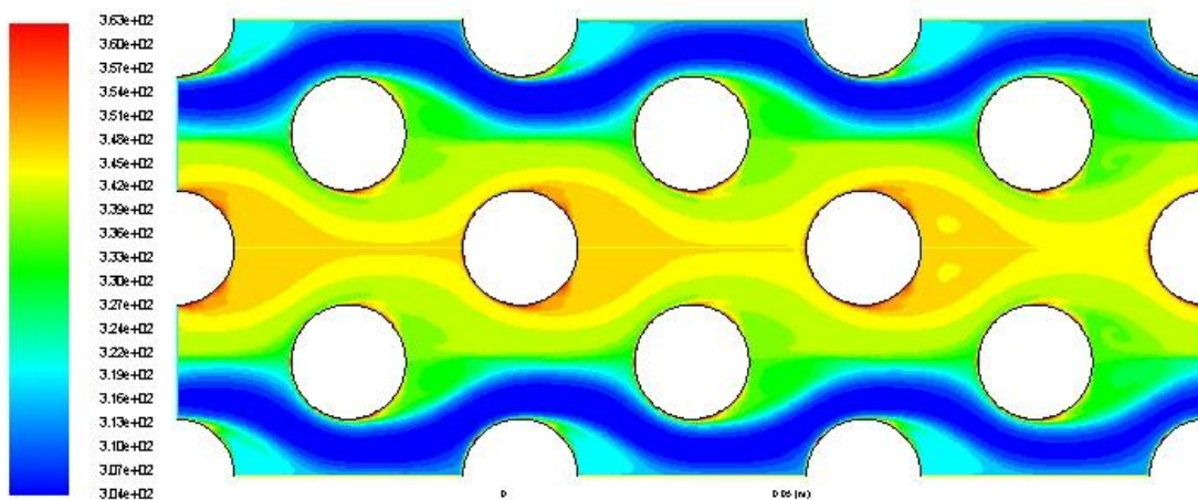
Figure IV.56 : contour de température concentration \phi=4\% et débit massique m=1\text{kg/s} (SiO 2 )
