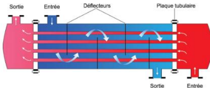
Figure II.8 : Le principe de fonctionnement
