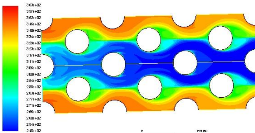
FigureIV.49 : contour de température pour concentration \text{Ø}=2\% et débit massique m=3\text{kg/s} (Cu)
