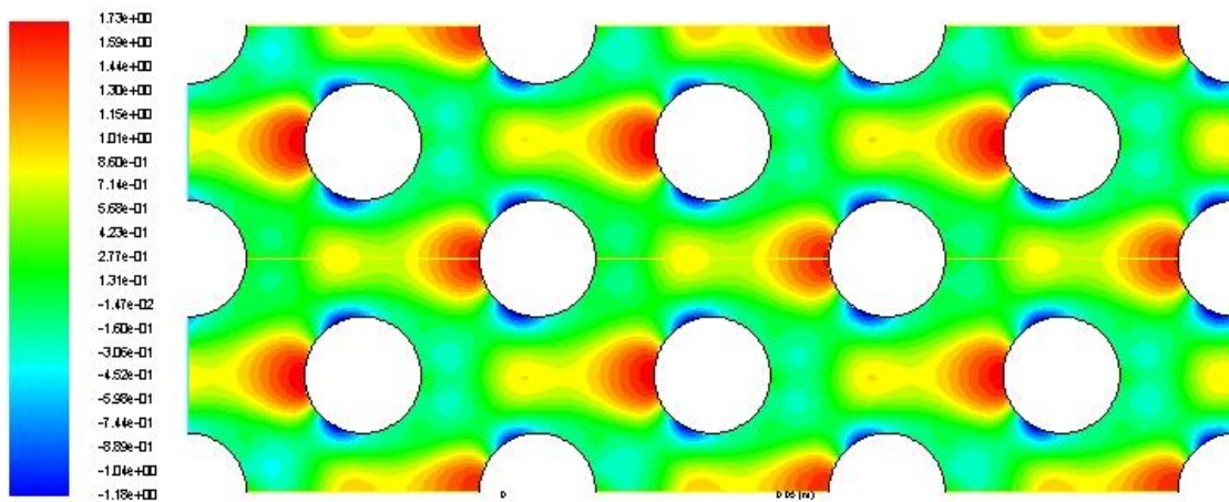
FigureIV.23 : contour de pression pour concentration \phi=1\% et débit massique m=1\text{kg/s} (SiO 2 )
