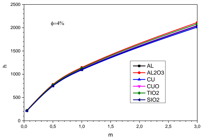
FigureIV.109 : Variation du coefficient de convection h (eau/nanofluides) en fonction de débit massique pour la concentration \Phi=4\%
