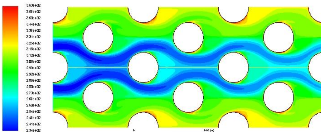
FigureIV.48 : contour de temperature pour concentration \text{Ø}=2\% et débit massique m=1\text{kg/s} (AL)
