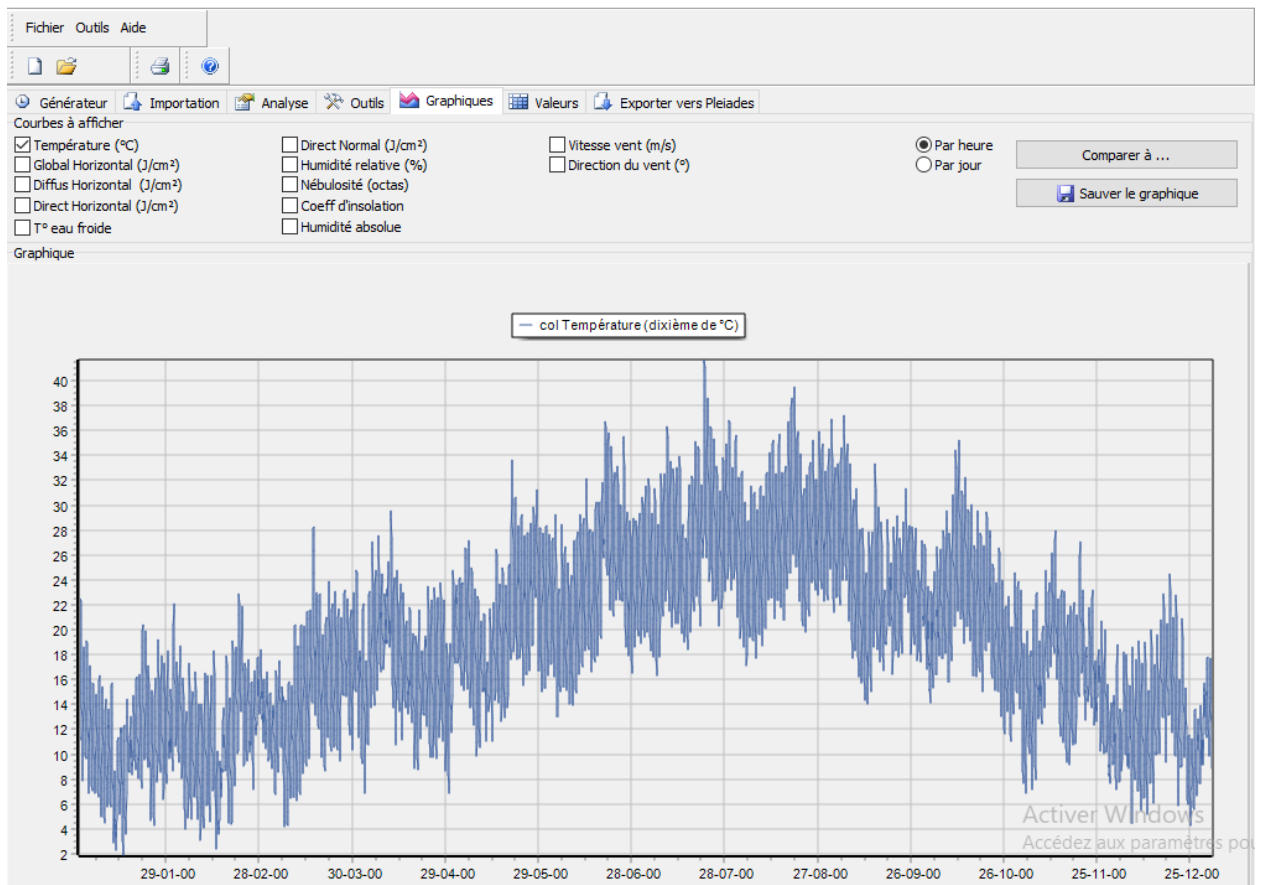
Figure 3-26 Température journalières maximales et minimales
