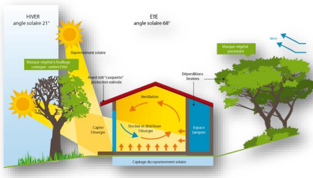
Figure 0-1 Schéma d'une habitation respectant les normes bioclimatiques.[5]
