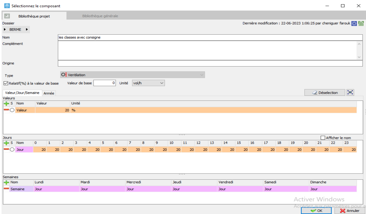
Figure 3-35 Scénario d'infiltration avec consigne de thermostat ( Les classes )
