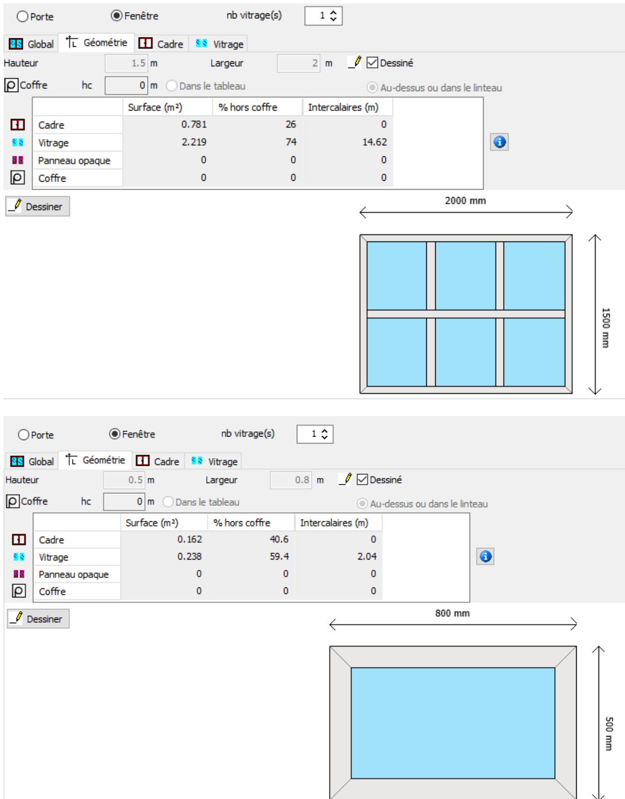
Figure 3-11 Caractéristique des Fenêtre en bois des classes
