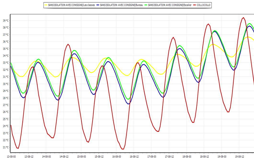
Figure 3-44 Evolution de la température de chaque zone pendant la semaine la plus chaud
