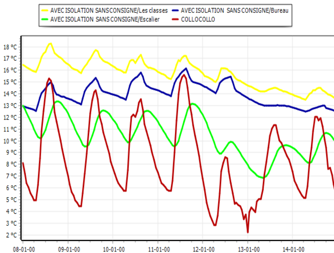
Figure 3-46 Evolution de la température de chaque zone pendant la semaine la plus froide
