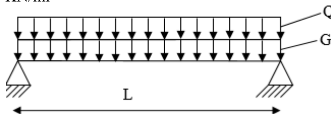
Figure III.16: Schéma statique d'une poutrelle isostatique
