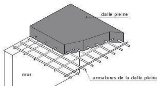
Figure II. 2 : Schéma du plancher à dalle pleine.
