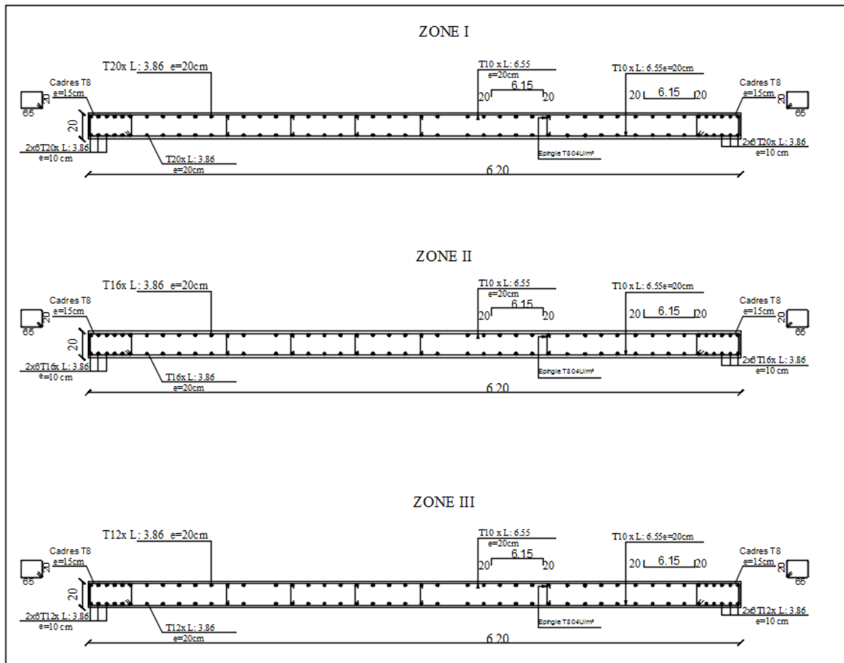
Schéma de Ferrailage des voiles V1 et V2
