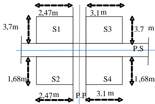
Figure II.9 : la surface reprise par le poteau central.
