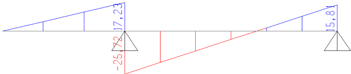
Figure III-13 Résultats des Efforts Tranchants trouvé avec SAP2000
