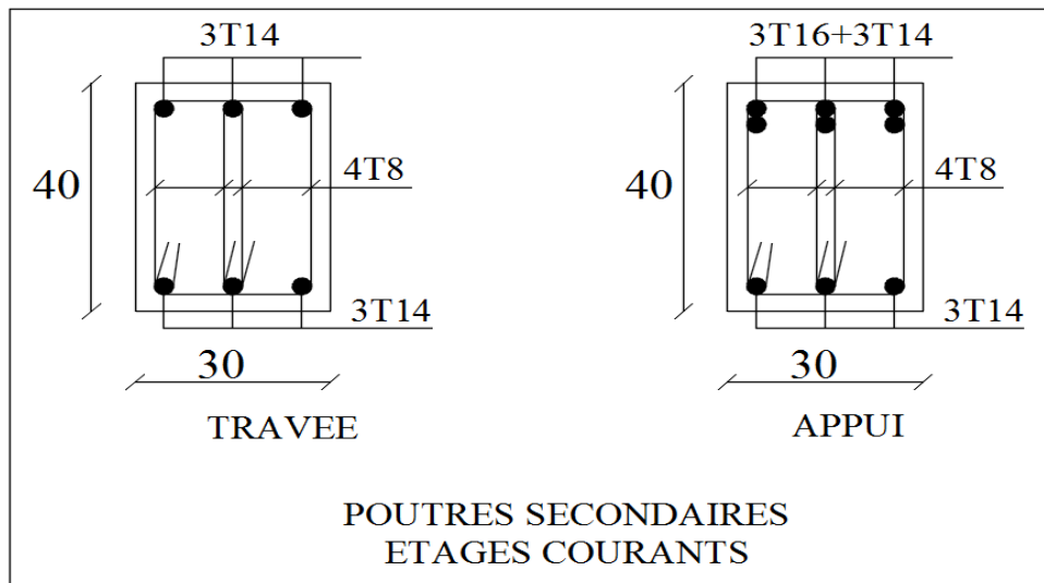
Figure V.5 : Ferraillage des poutres secondaires
