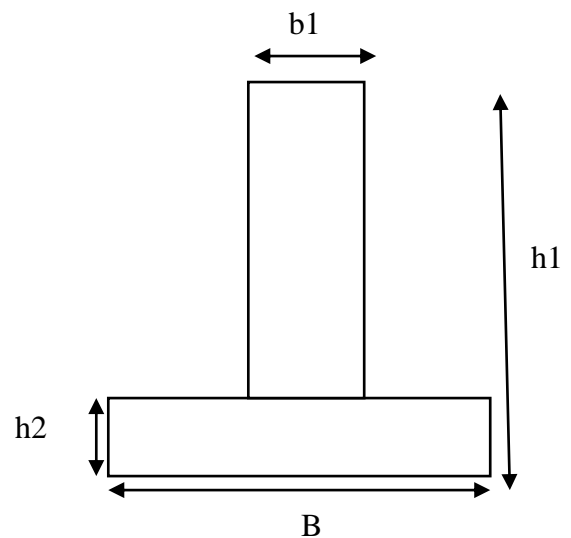
Figure VI.7 : Semelle filante forme « T ».
