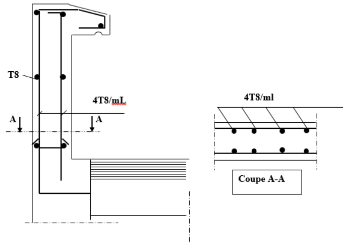
Figure III-4 Ferrailage de l'acrotère
