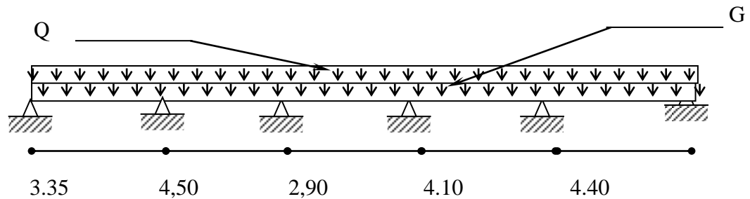
Figure III.16: schéma statique de la poutrelle à plusieurs travées III.5.1.1.1 Détermination des efforts internes :
