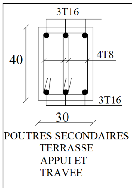
Figure V.6 : Ferraillage des poutres secondaires
