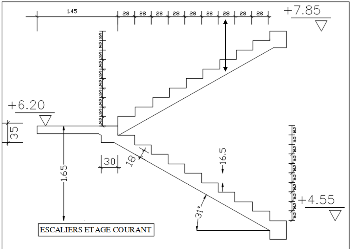
Figure III.8 : Schéma statique de l'escalier
