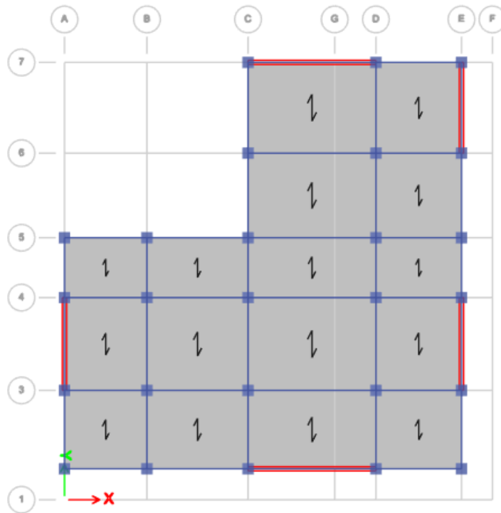
Figure V.6 : Plan de repérage des voiles.
