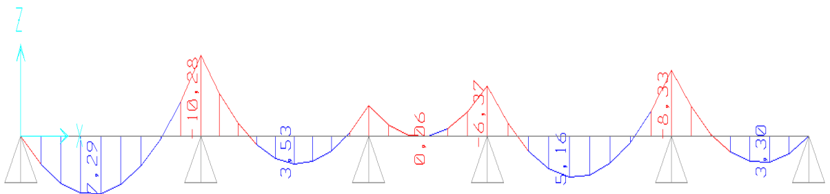
Figure III.19 Moments ELS
