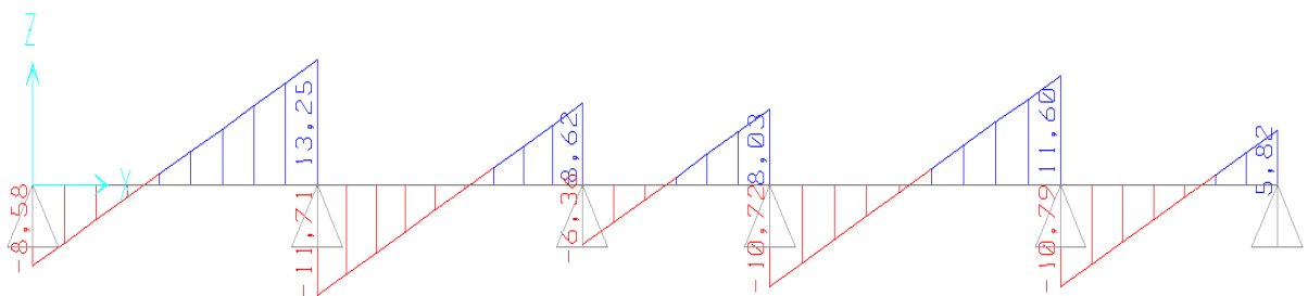
Figure III.20 Efforts Tranchants ELS
