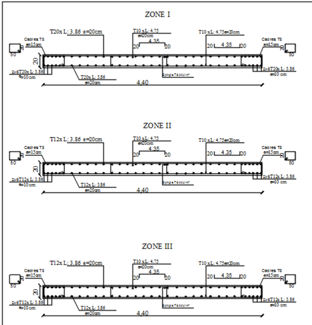
Schéma de Ferrailage des voiles V5
