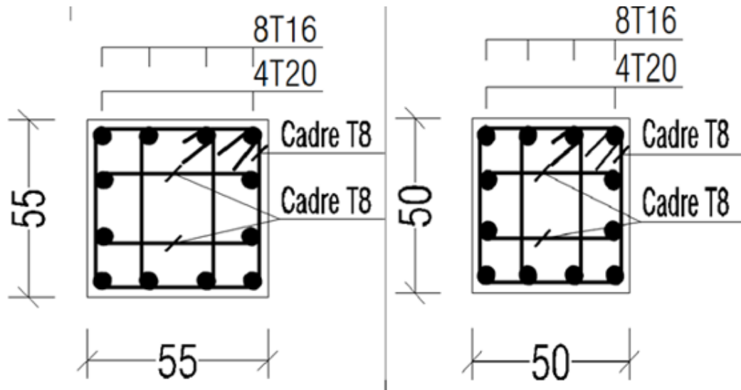
FigureV.1 : Schéma de ferrailage des poteaux.
