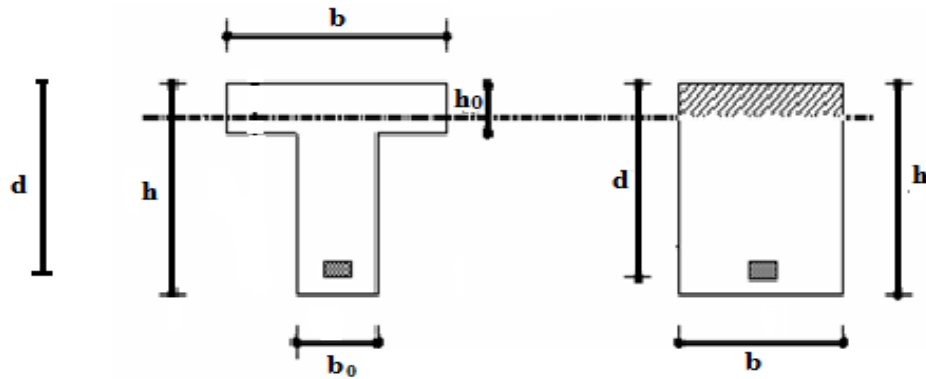
Figure III.17 : Section rectangulaire et section en “Té” en travée.
