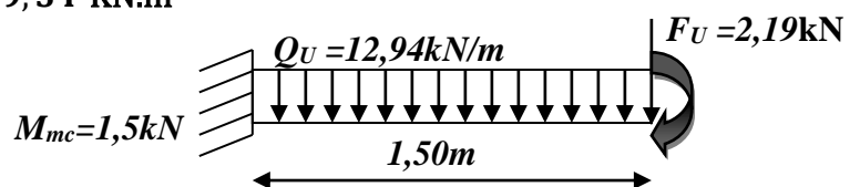
Figure III-6 Schéma statique du balcon
