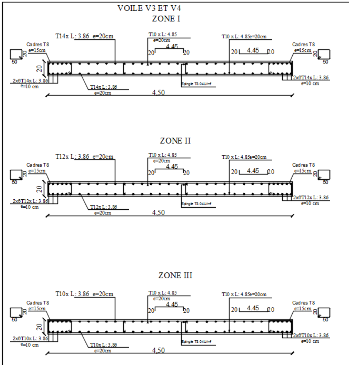
Schéma de Ferrailage des voiles V3 et V4
