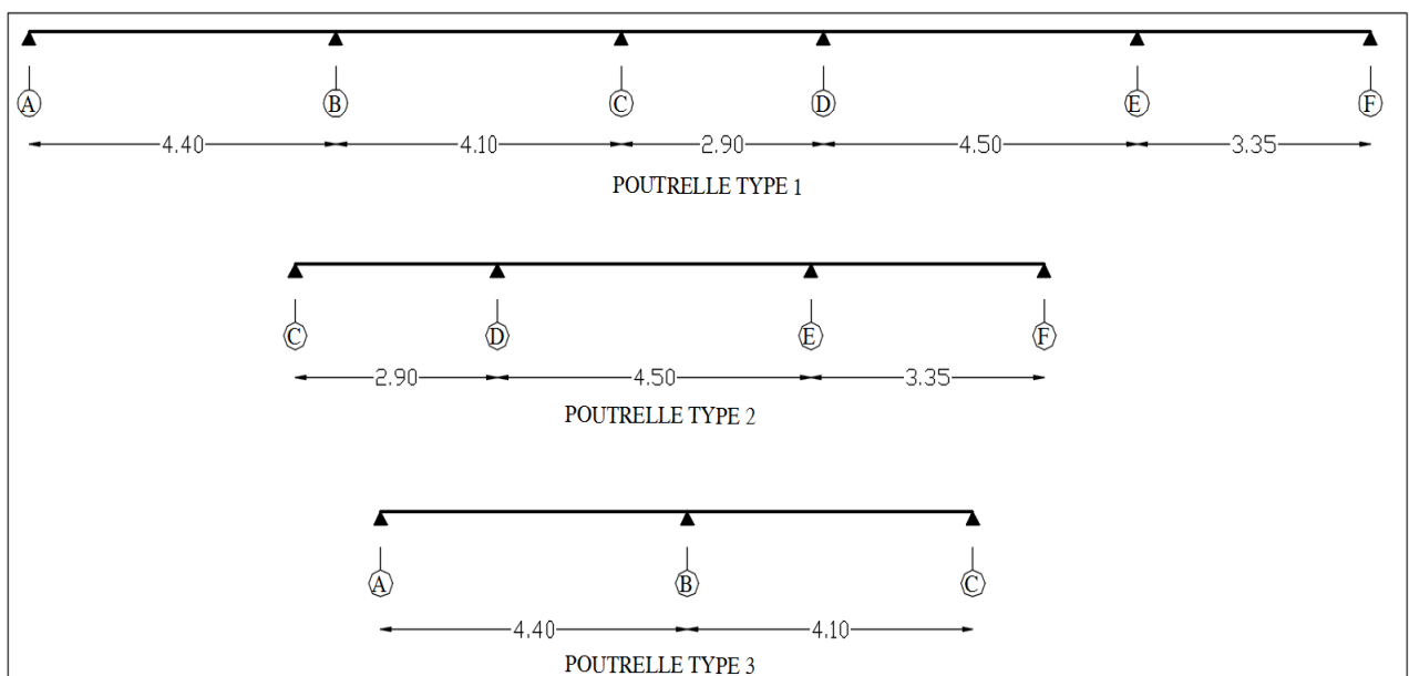
Figure III-15 Types de poutrelles
