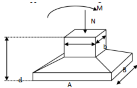
Figure VI. 5 : Semelles isolée sous poteaux.
