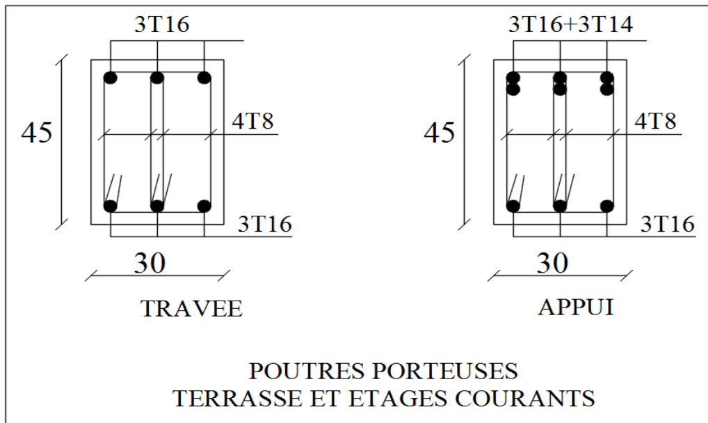
Figure V.3 : Ferrailage des poutres principales
