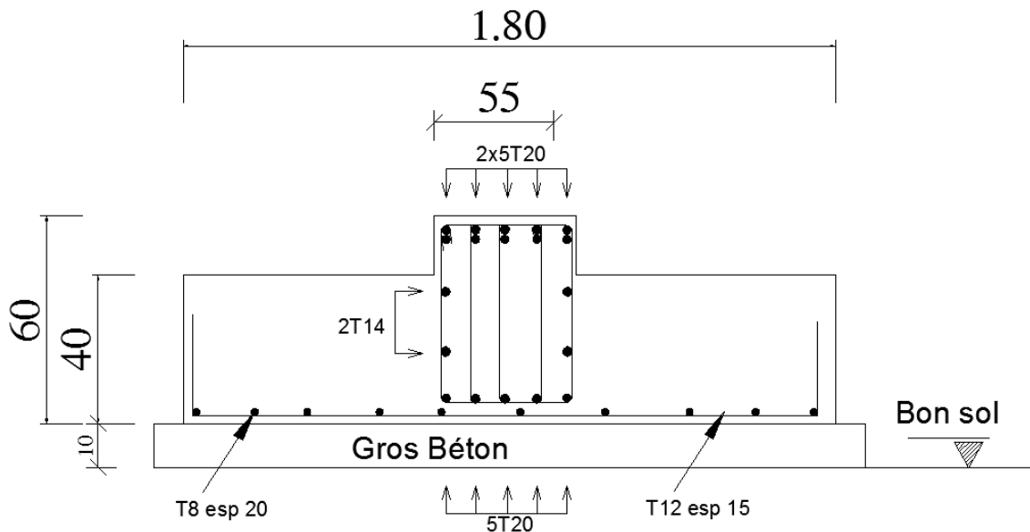
Figure VI.9 : Schéma de ferrailage de la semelle et la nervure.
