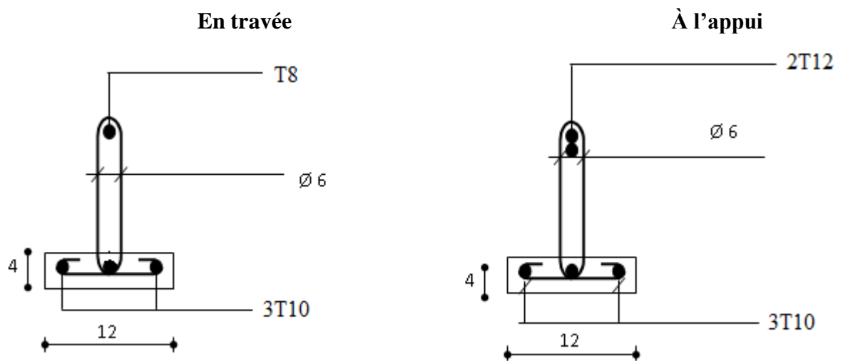
Figure III.18 : Ferrailage des poutrelles sur les différents étages
