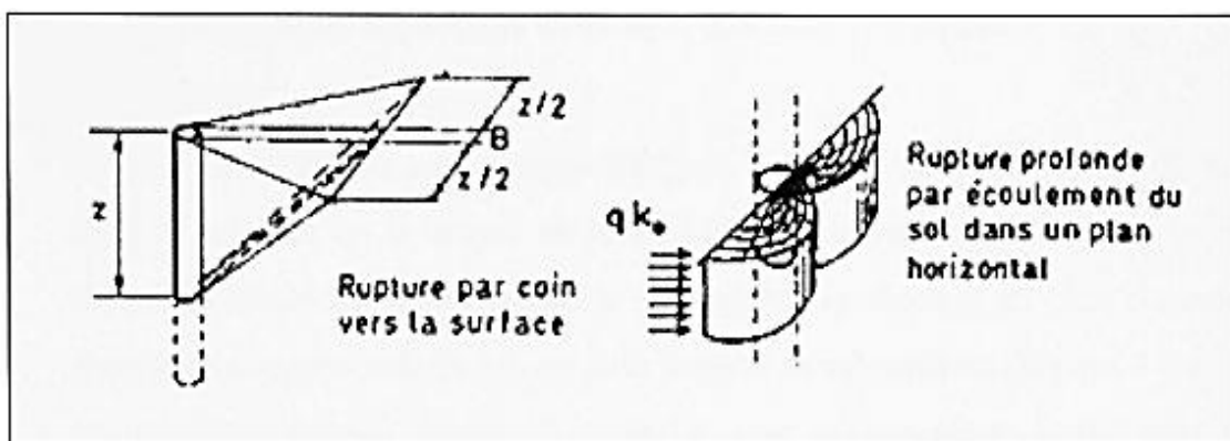
Figure B.3 : Mécanismes de rupture selon Blum et Brinch- Hansen. (Tiré de Bague linet Gézéquel, 1972). [1]
