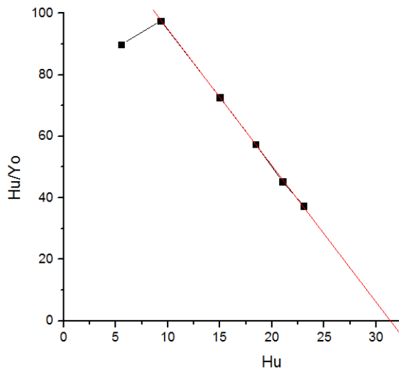
Figure 4.9 : critère Décourt.
