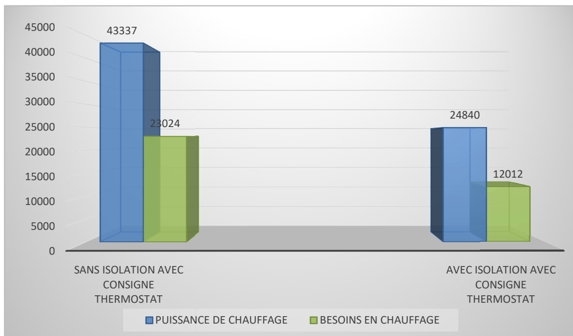
Figure : Histogramme de Besoin en Chauffage et puissance de chauffage pour les deux variantes
