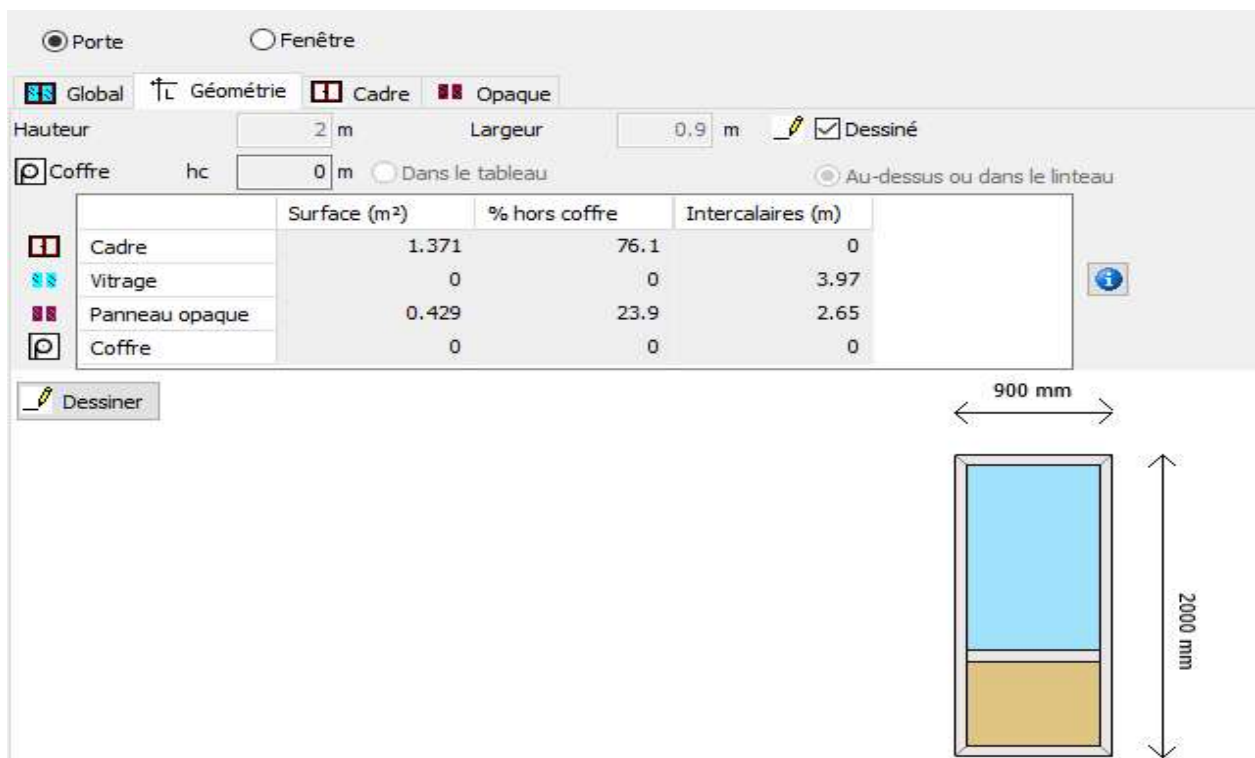
Figure 3-13 Caractéristique de porte en PVC du Bureau
