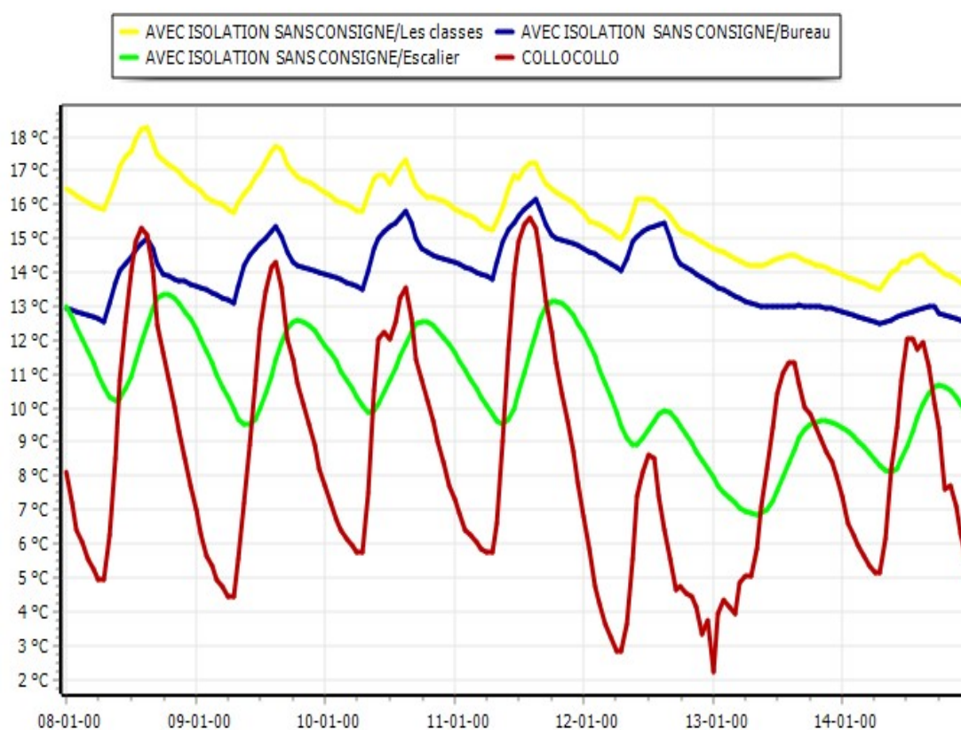
Figure 3-46 Evolution de la température de chaque zone pendant la semaine la plus froide
