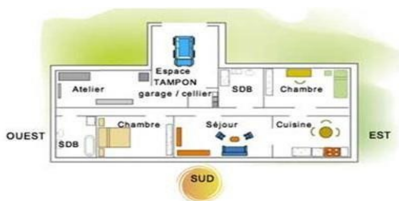
Figure 0-7 la distribution des espaces dans une maison bioclimatique.
