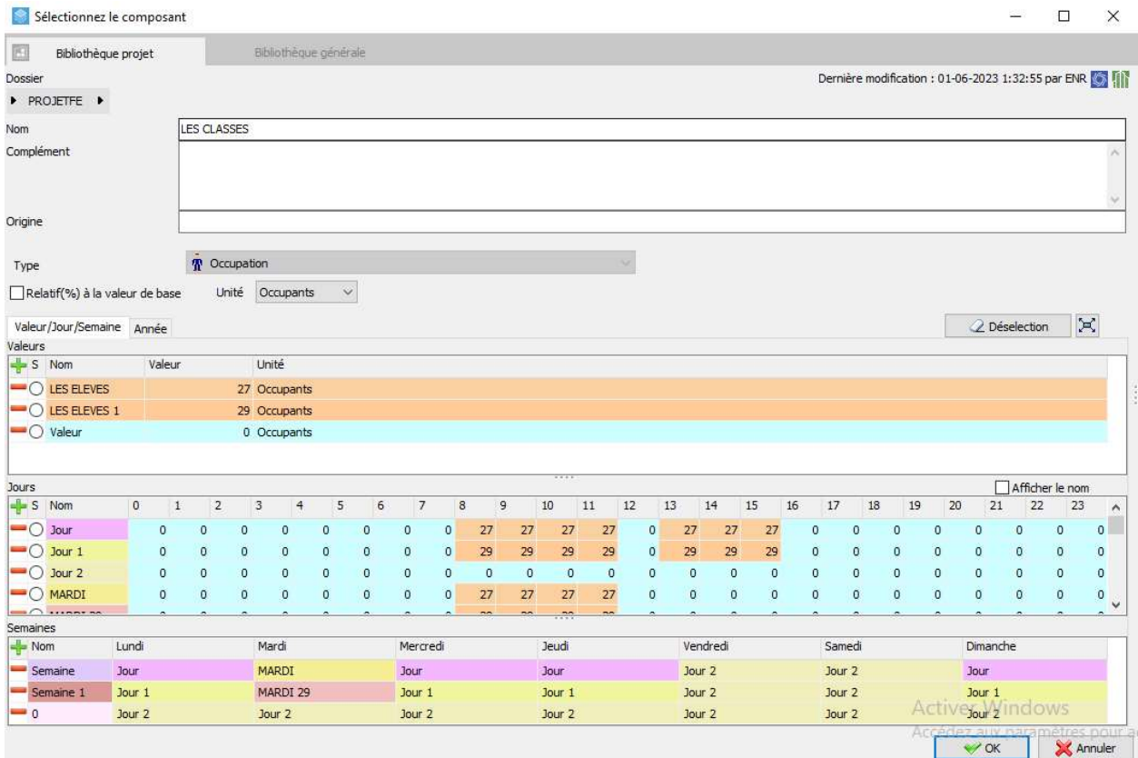
Figure 3-28 Scénario d'occupation pour la 1 ère zone
