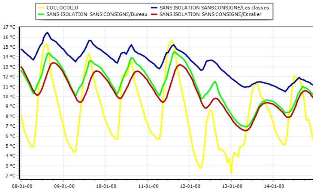
Figure 3-41 Evolution de la température de chaque zone pendant la semaine la plus froid
