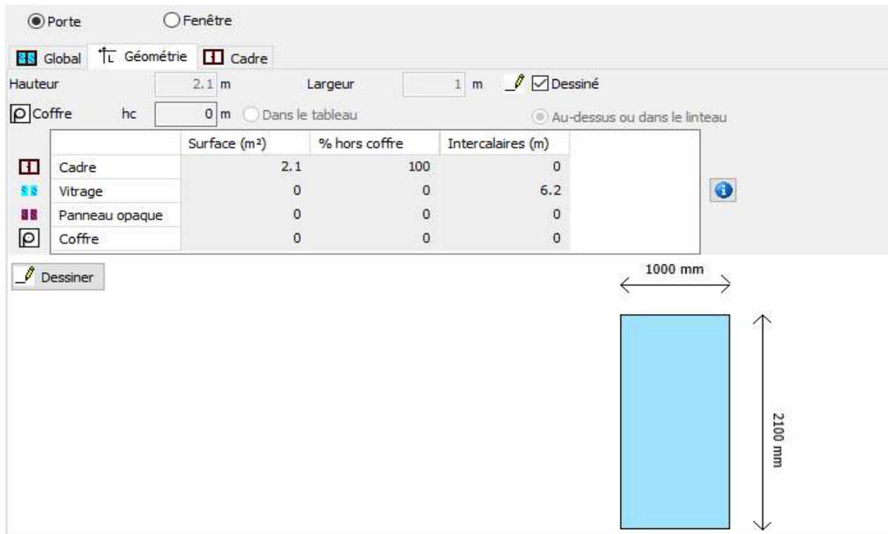
Figure 3-12 Caractéristique des portes en bois des classes
