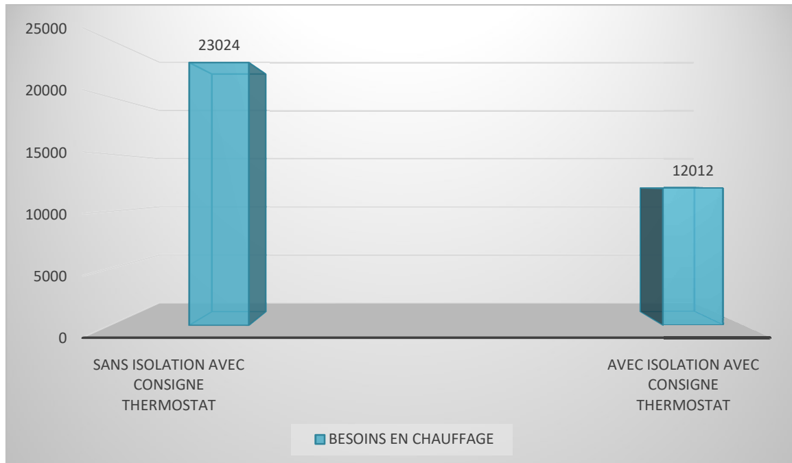
Figure : Histogramme des Besoins en Chauffage pour les deux variantes
