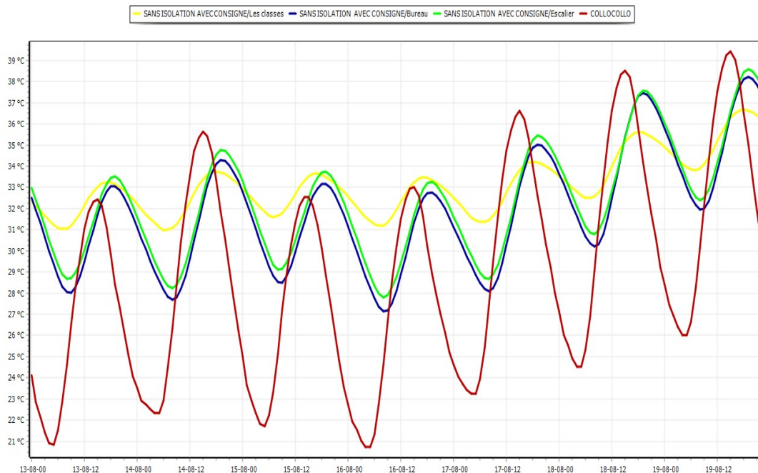
Figure 3-44 Evolution de la température de chaque zone pendant la semaine la plus chaud
