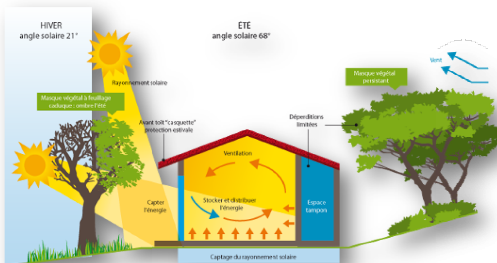
Figure 0-1 Schéma d'une habitation respectant les normes bioclimatiques.[5]
