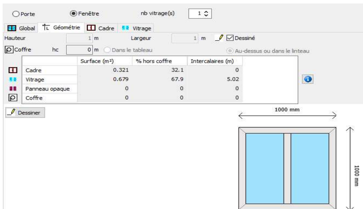
Figure 3-10 caractéristique de Fenêtre PVC pour Bureau
