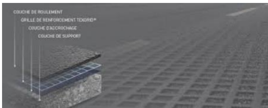
Figure II.12 : Géotextile-géo grille
