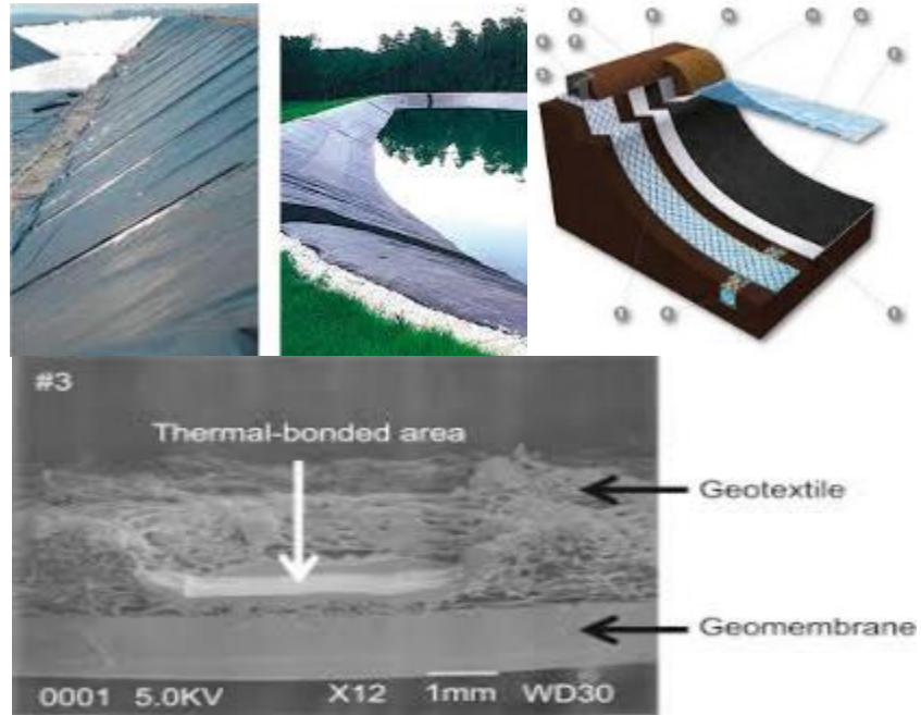
Figure II.11 : géotextile-géo membrane
