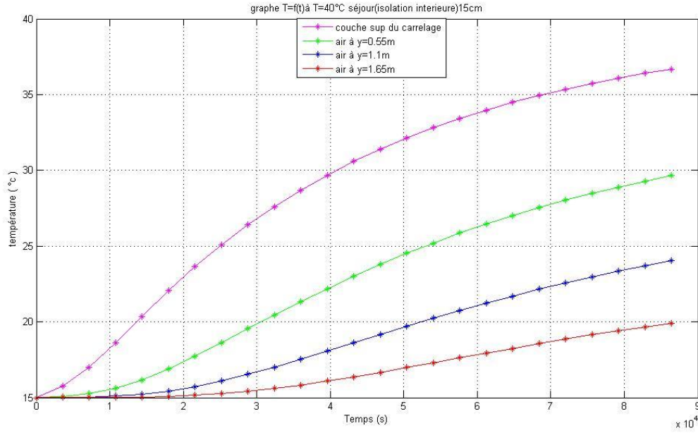
Figure4.32 évolution de la température en fonction du temps (isolation intérieure)séjour e= 15 cm (24h)
