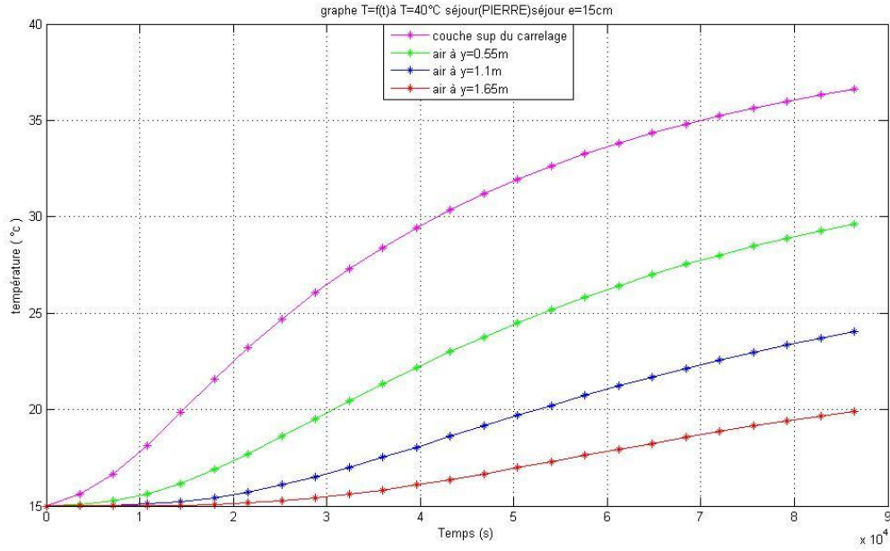
Figure4.45 évolution de la température en fonction du temps (PIERRE)Séjour e= 15cm (24h)
