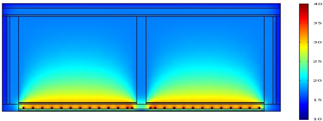
Figure 4.7. Résultat pour un temps de 15h coupe1.
