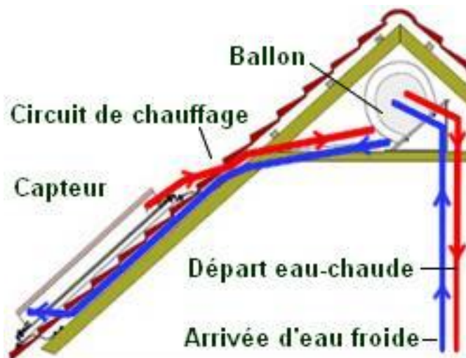
Figure.1.2 Principe de chauffe eau thermosiphon[13]
