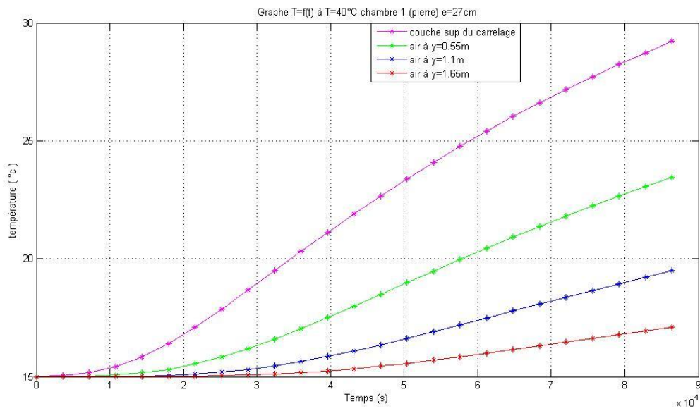
Figure4.46 évolution de la température en fonction du temps (PIERRE)Chambre 1 (24h) e=27cm
