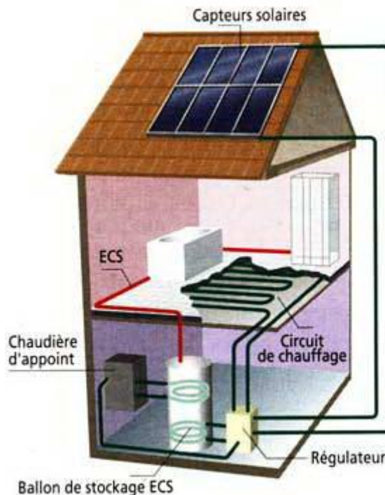
Figure. 1.6 Schéma d'une installation de chauffage solaire par le plancher et l'eau chaude sanitaire[14]
