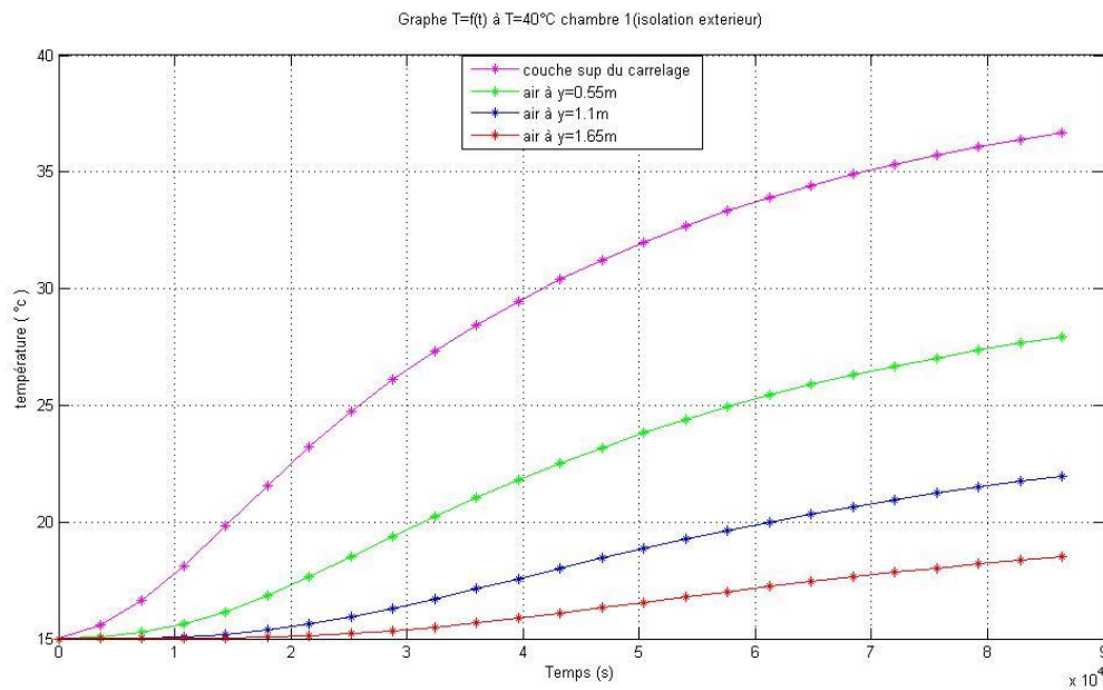
Figure 4.35 évolution de la température en fonction du temps (isolation extérieure) chambre 1
