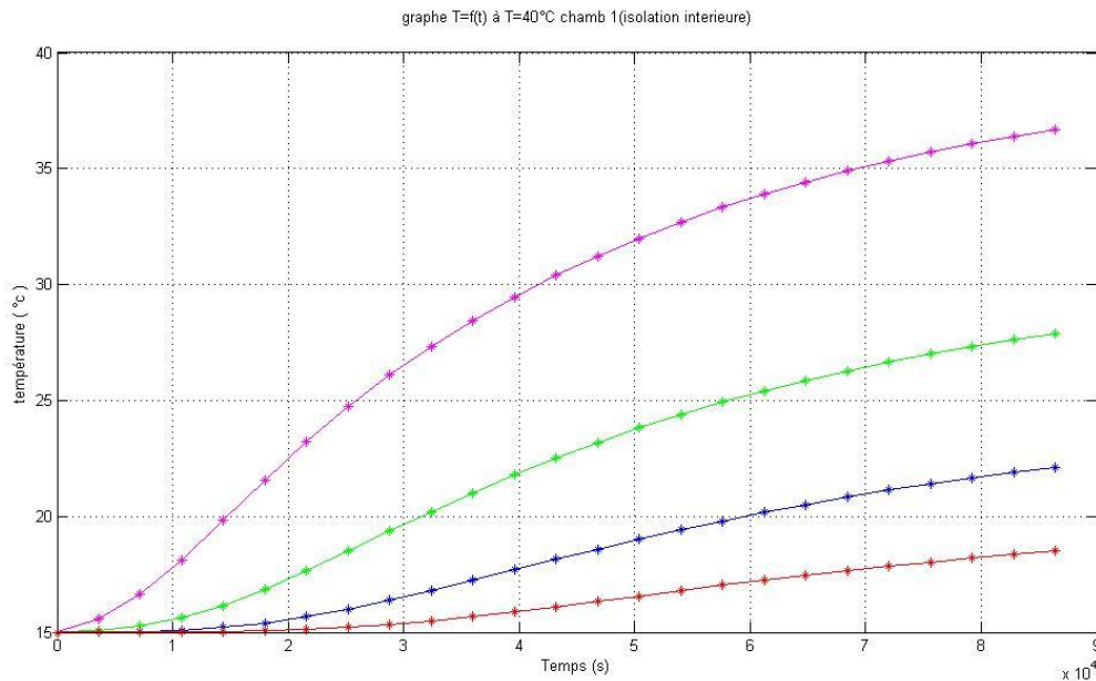
Figure 4.31 : évolution de la température en fonction du temps (isolation intérieure)chambre 1 e= 15 cm (24h)
