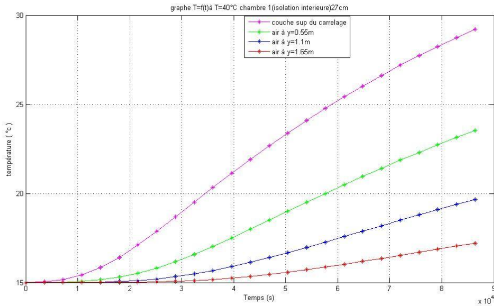
Figure4.33 évolution de la température en fonction du temps (isolation intérieure)chambre 1 e= 27 cm (24h)
