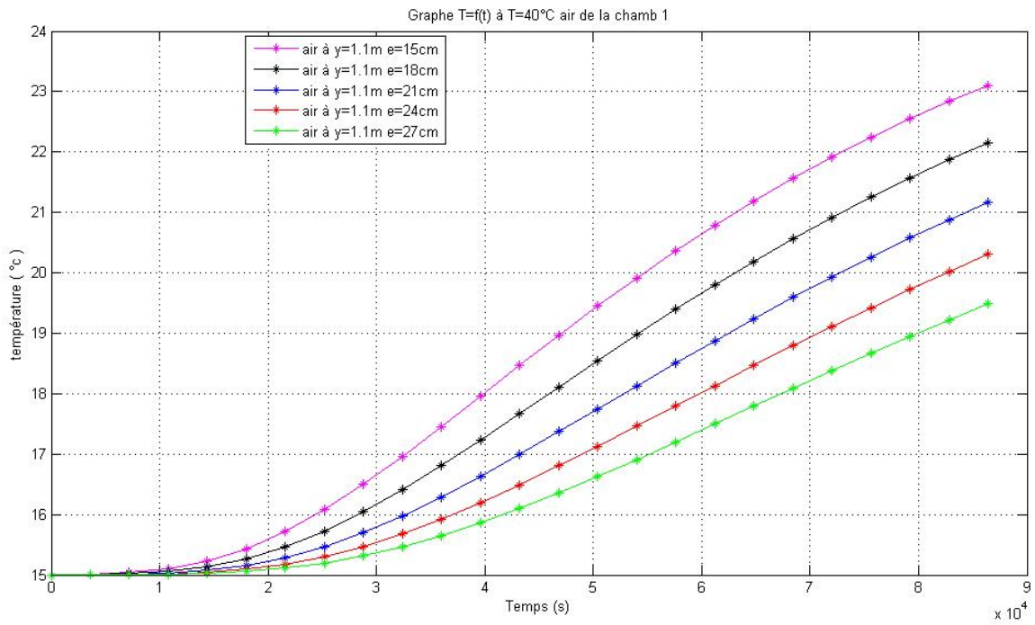
Figure 4.17 Evolution de la température en fonction du temps air 2 de la chambre 1(24h)
