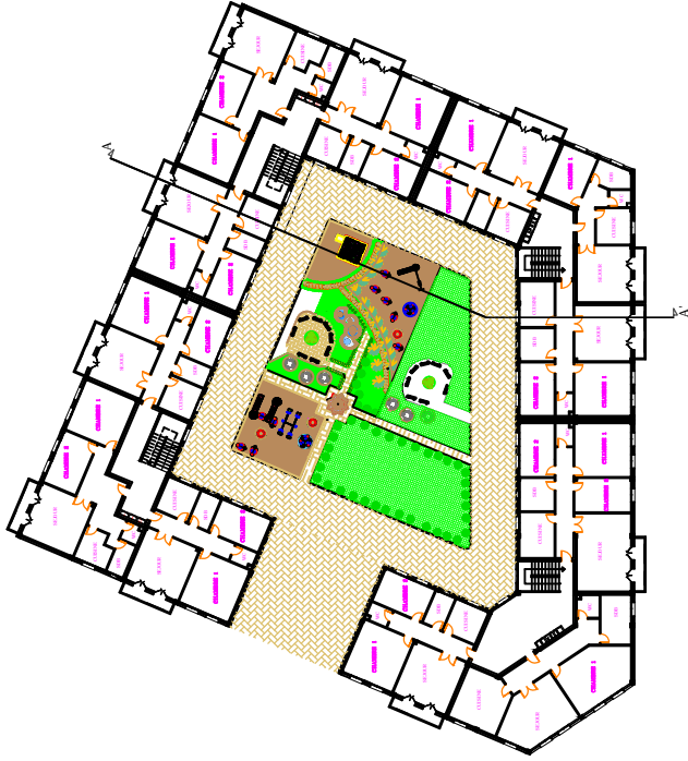
PLAN DES ETAGE
