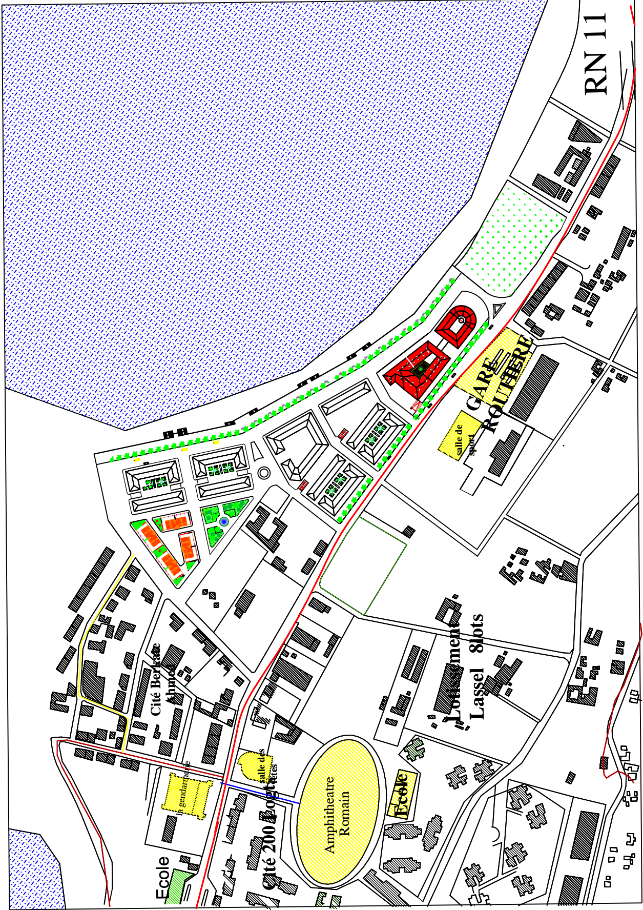
PLAN DE MASSE
