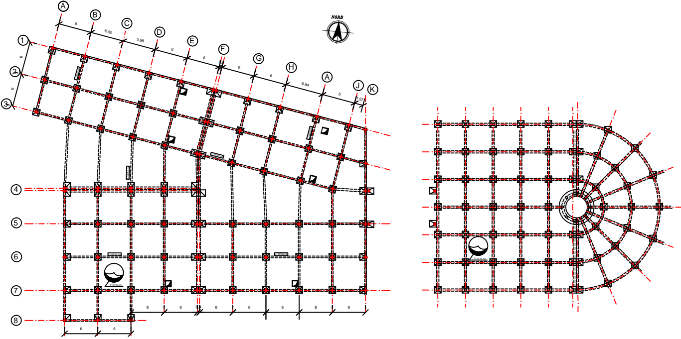
PLAN FONDATION
