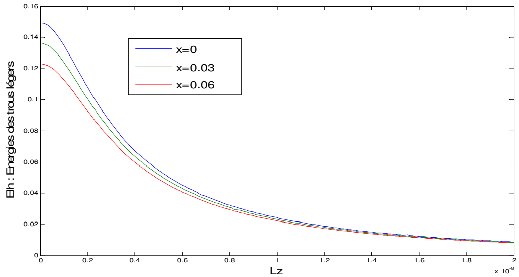
Figure III-18 : Evolution des énergies de confinement des trous légers en fonction de l'épaisseur du puits quantique L_z
