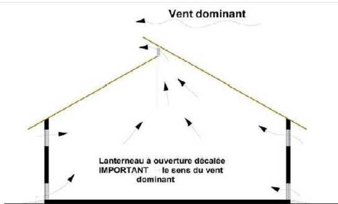
Figure5 : Lanterneau à ouverture décalée (Djago et al.2007a).
